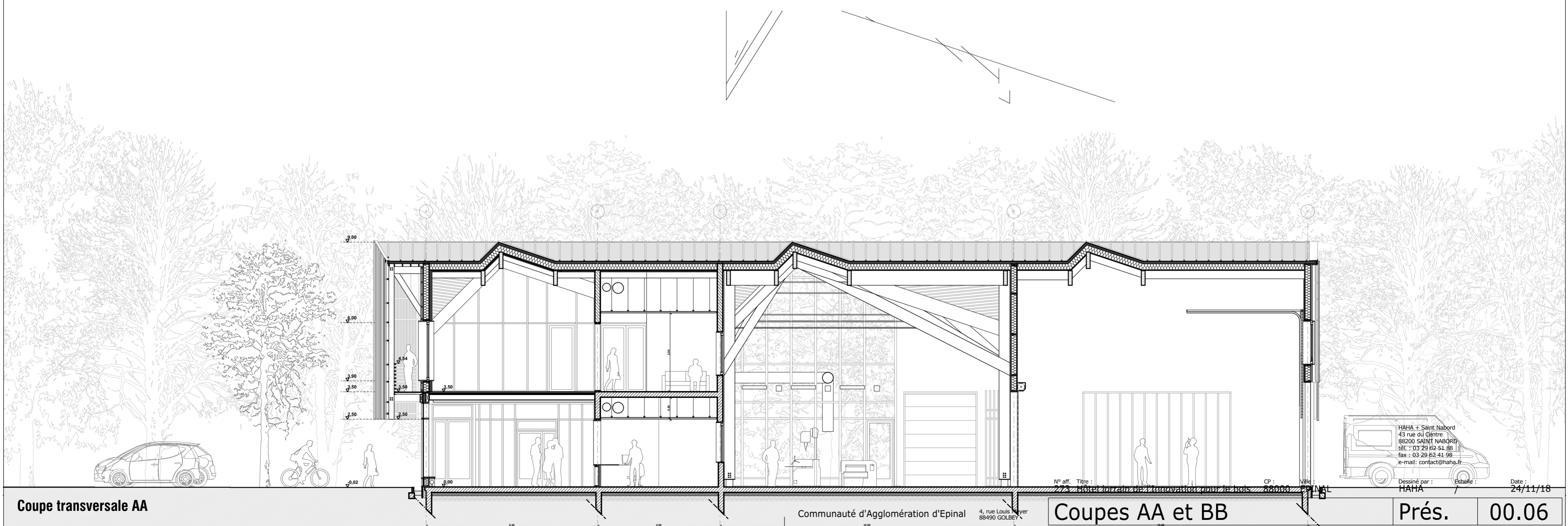
Coupe longitudinale BB
