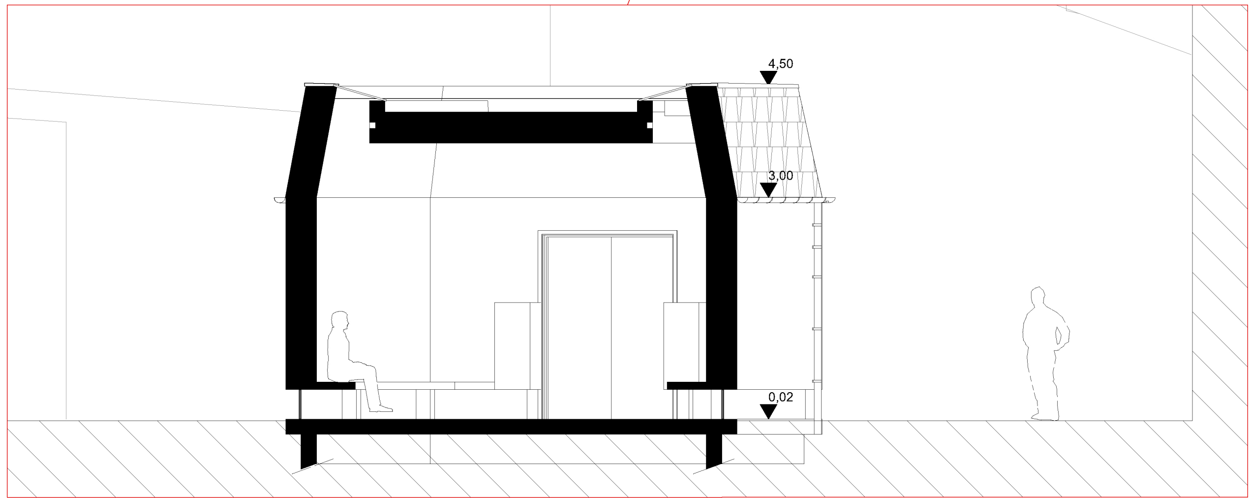
Coupe DD
