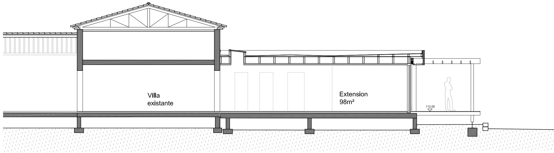
Coupe longitudinale
