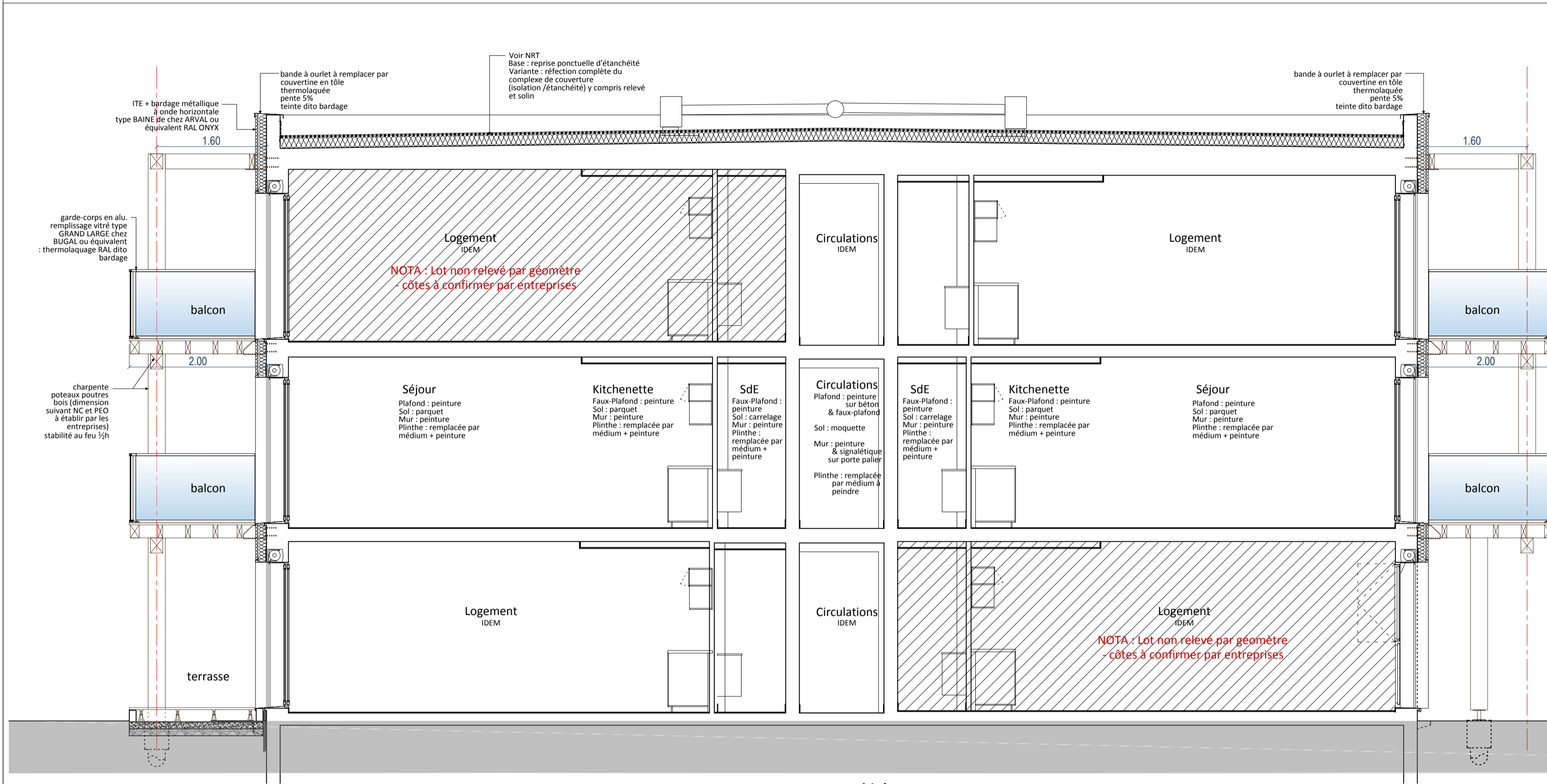
Coupe 1-1' bât. B
