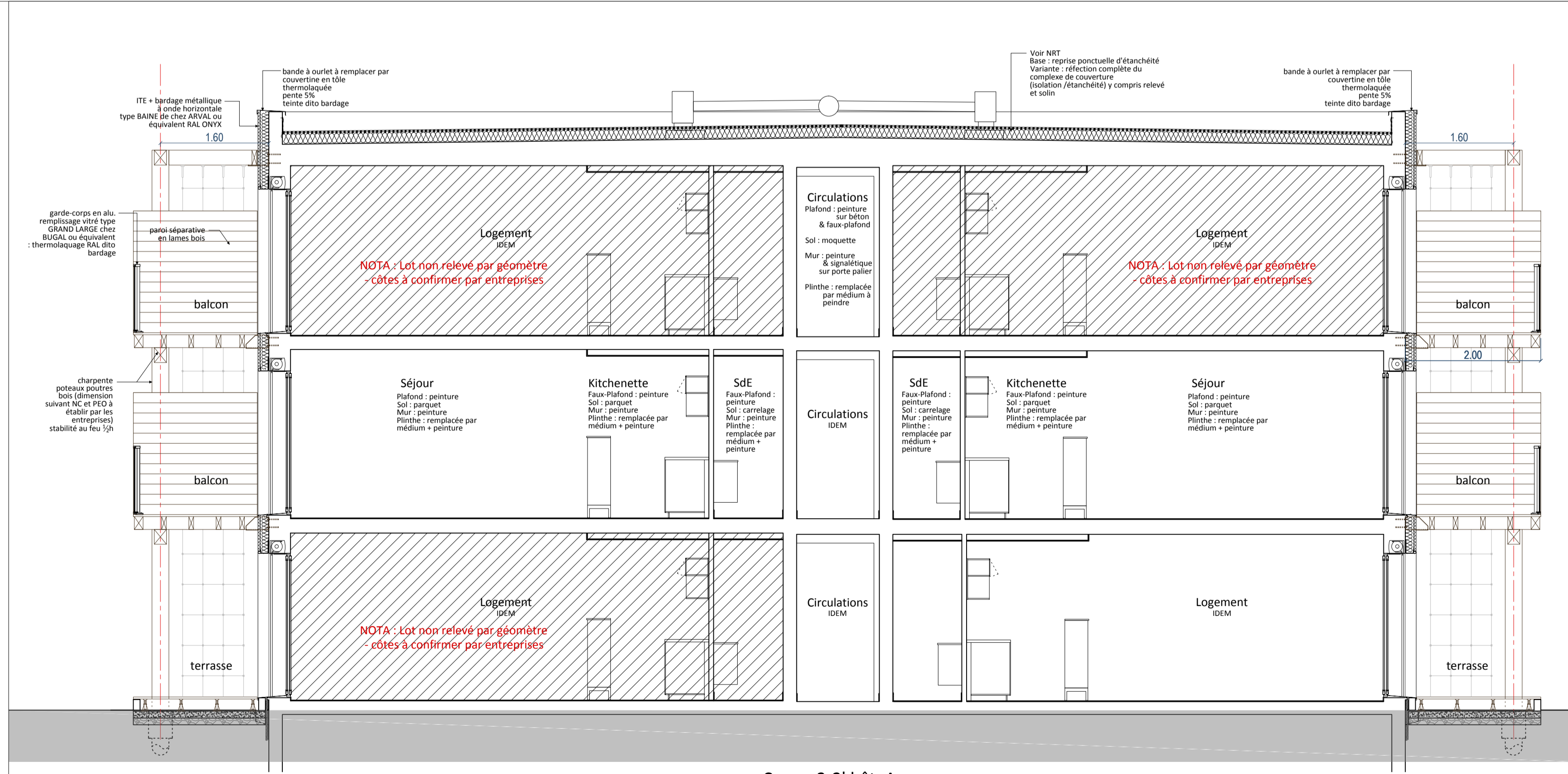
Coupe 2-2' bât. A
