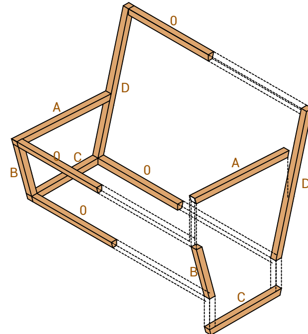
Eclaté Assise 1
