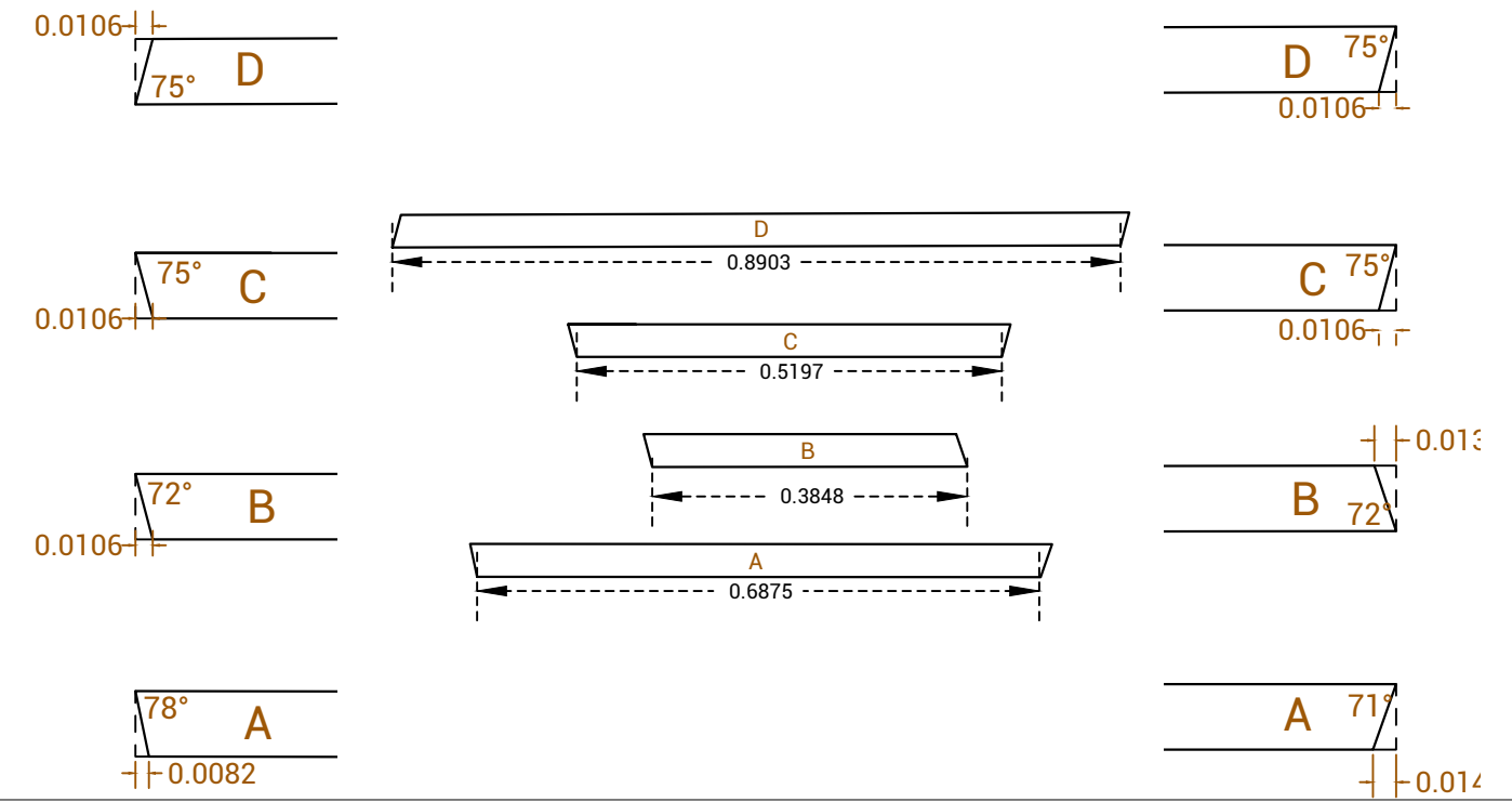
Détail section des profils Assise 1
