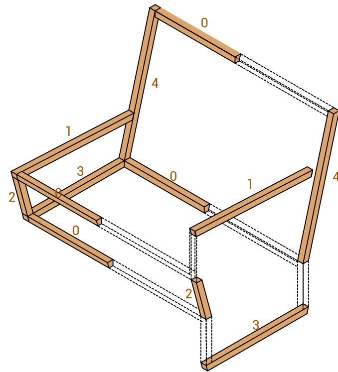
Eclaté Assise 2
