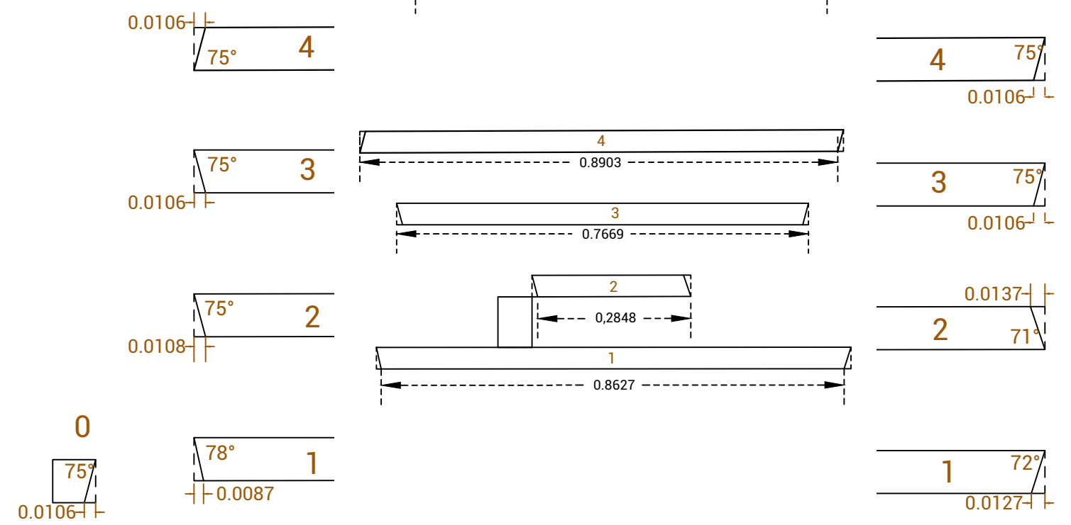
Détail section des profils Assise 2
