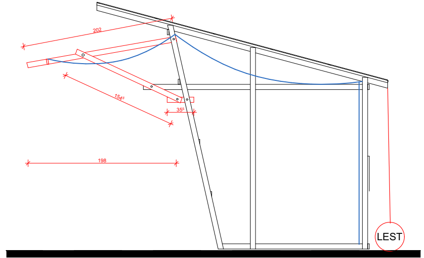
Elevation laterale
