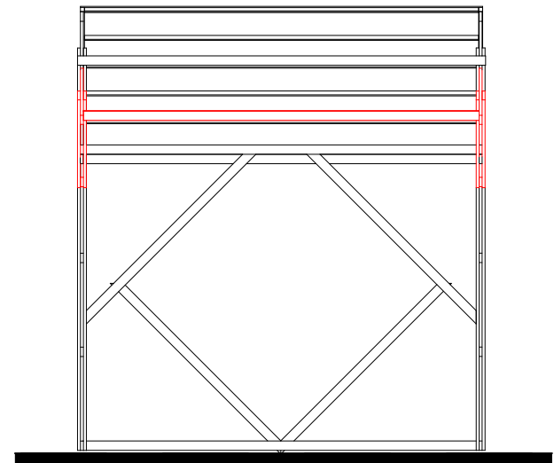
Elevation longitudinale
