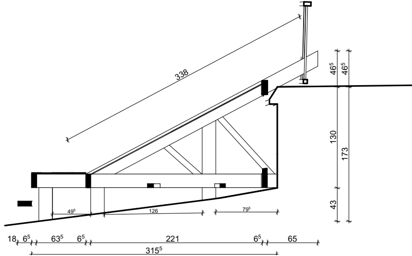
COUPE C 23
