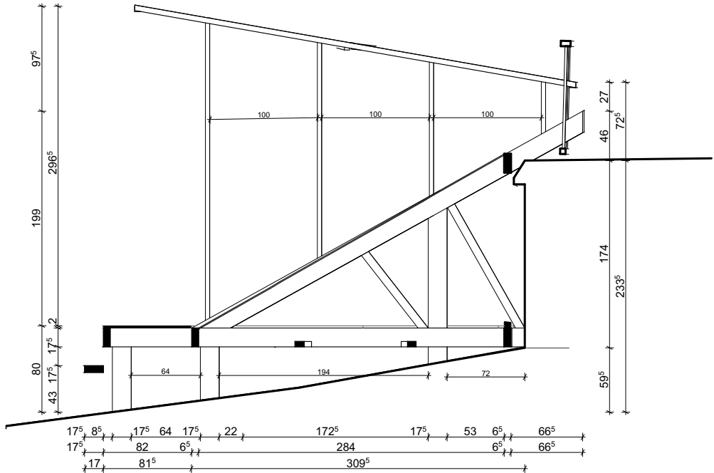
COUPE C 25
