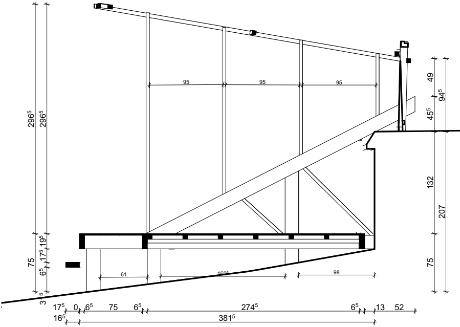
COUPE C 24
