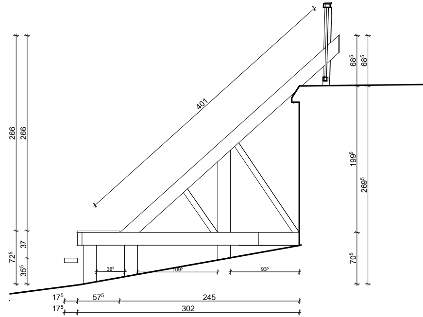
COUPE C 27
