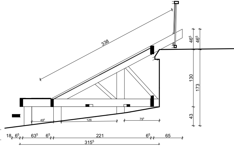
COUPE C 23
