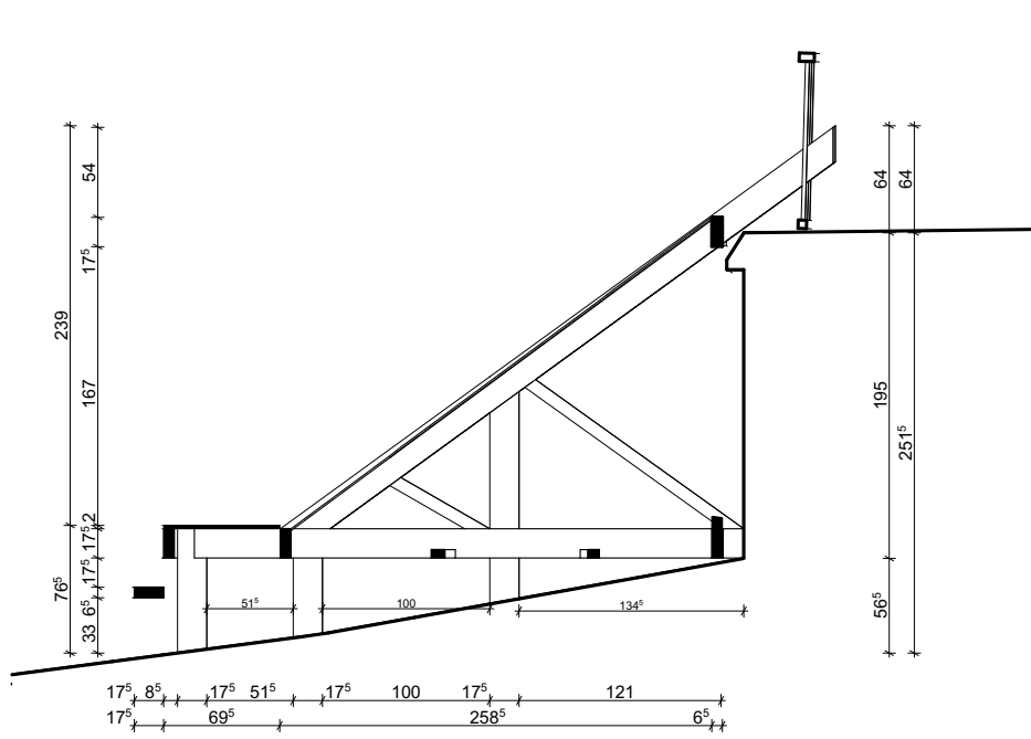
COUPE C 26
