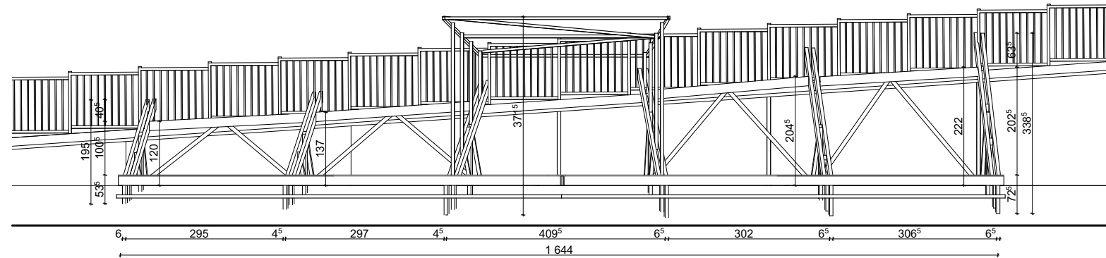
COUPE C 28
