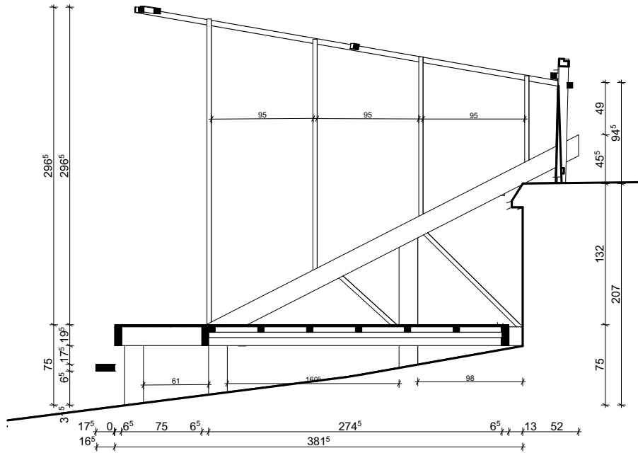
COUPE C 24
