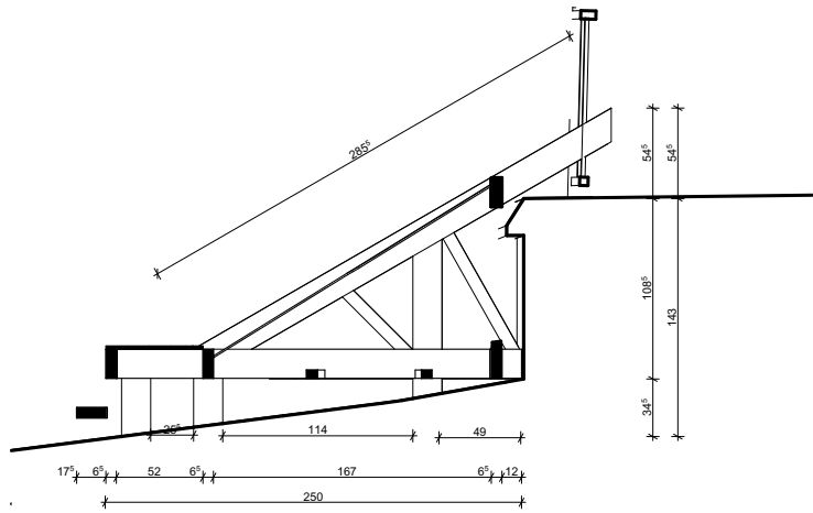
COUPE C 22
