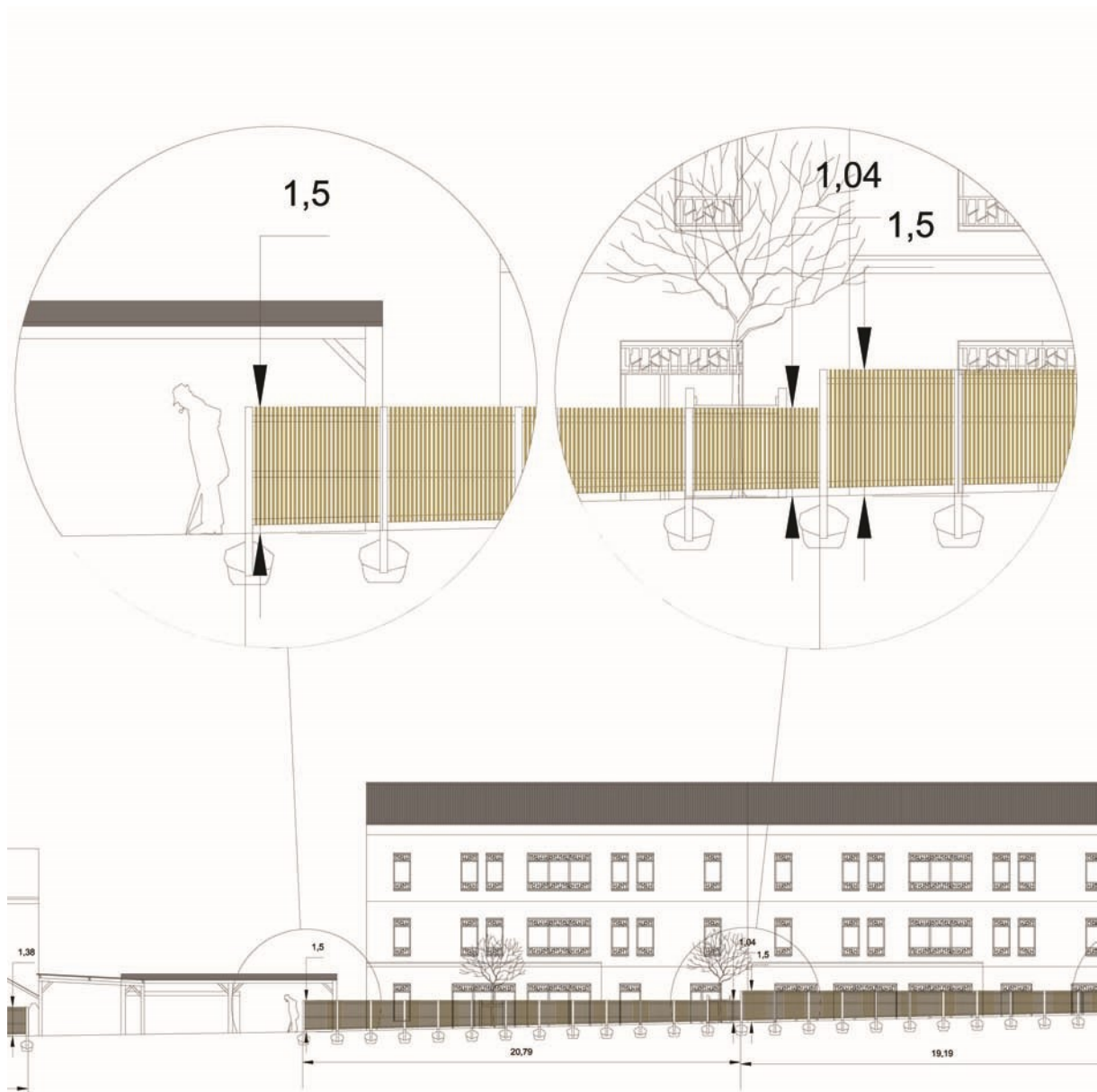
Coupe clôture façade Ouest
