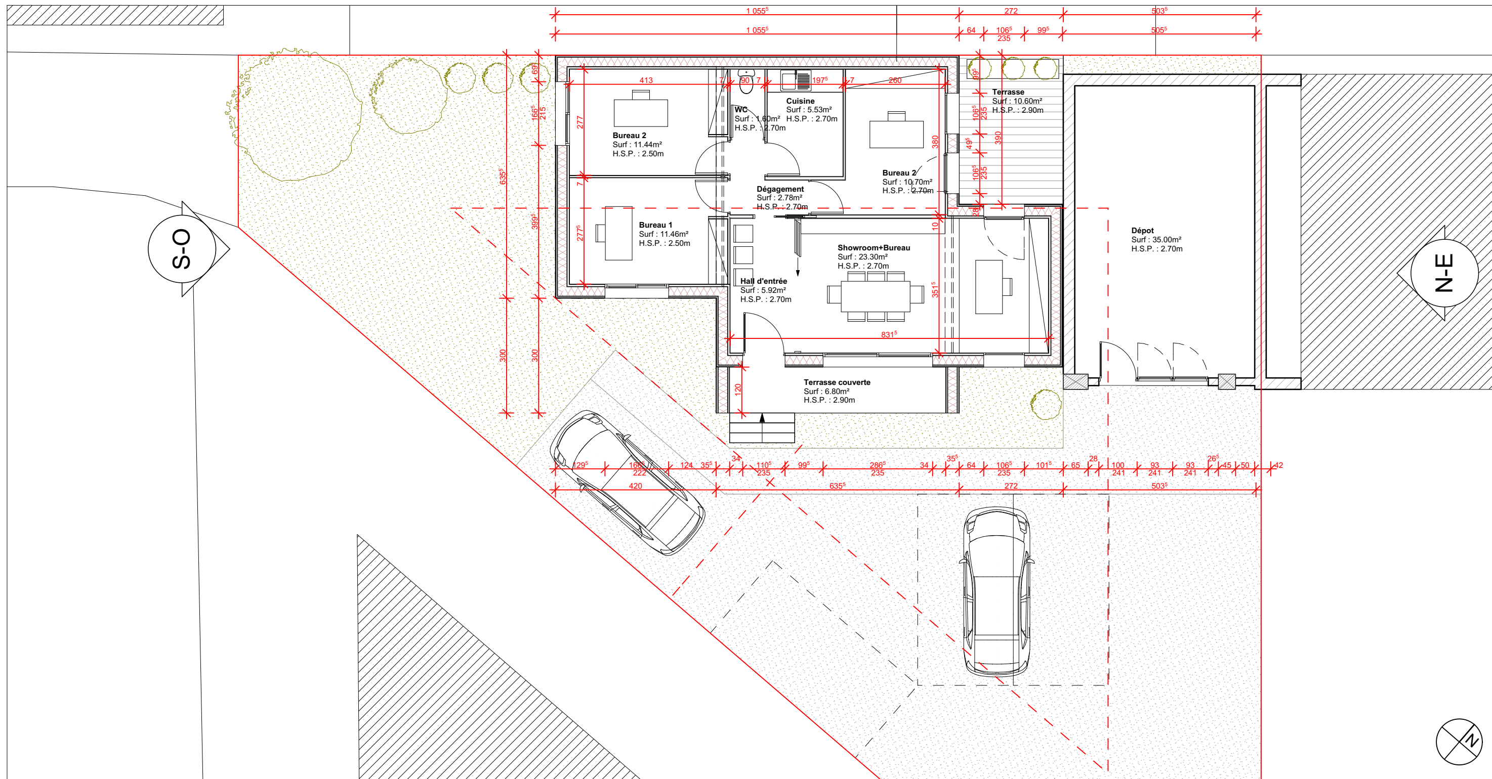
Plan RDC 1/100
