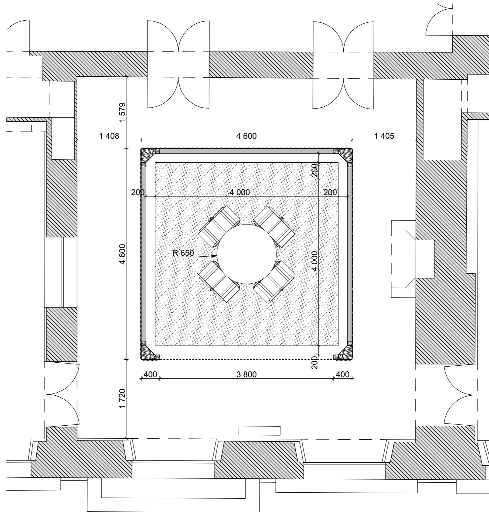
PLAN ECHELLE 1/50
