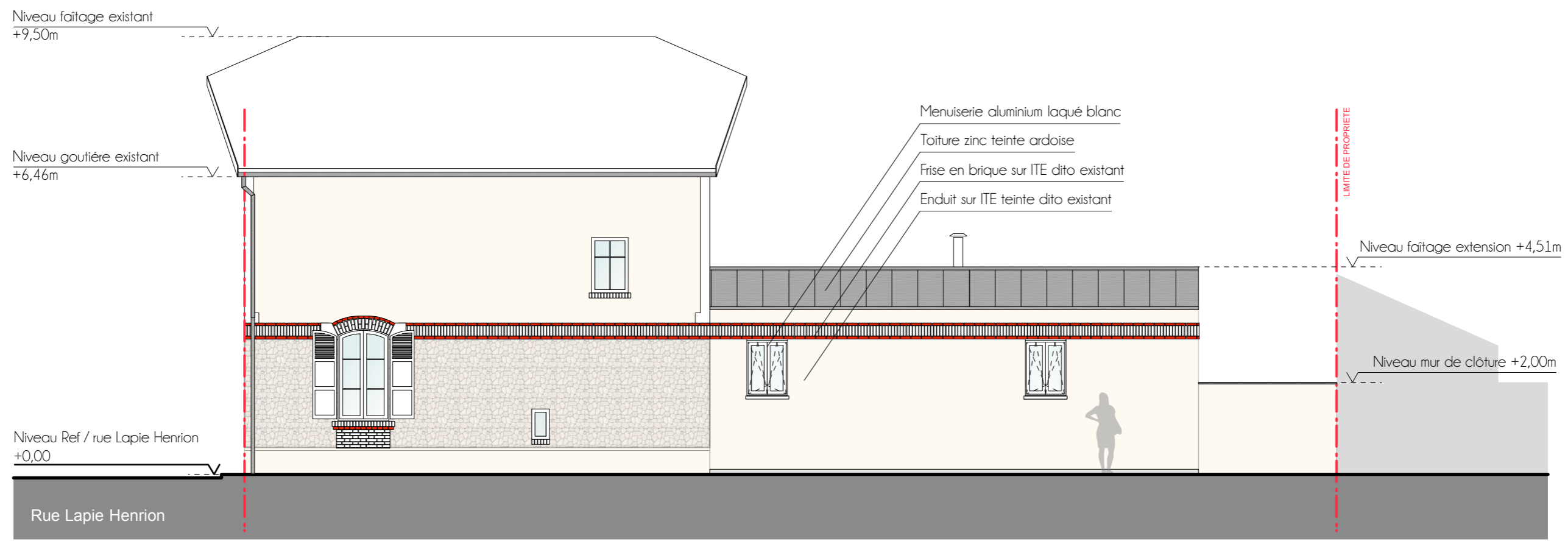
PC5 - FACADE SUR LA RUE DE NORMANDIE
