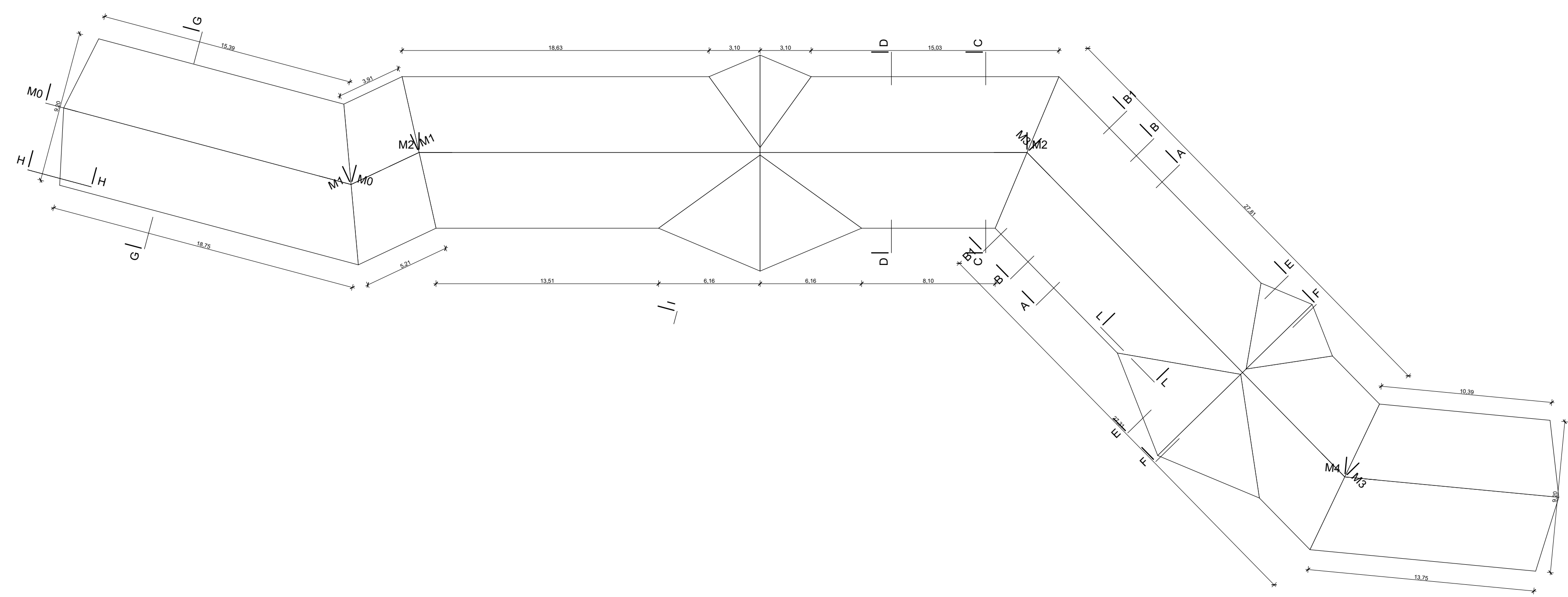
Couverture 1/200
