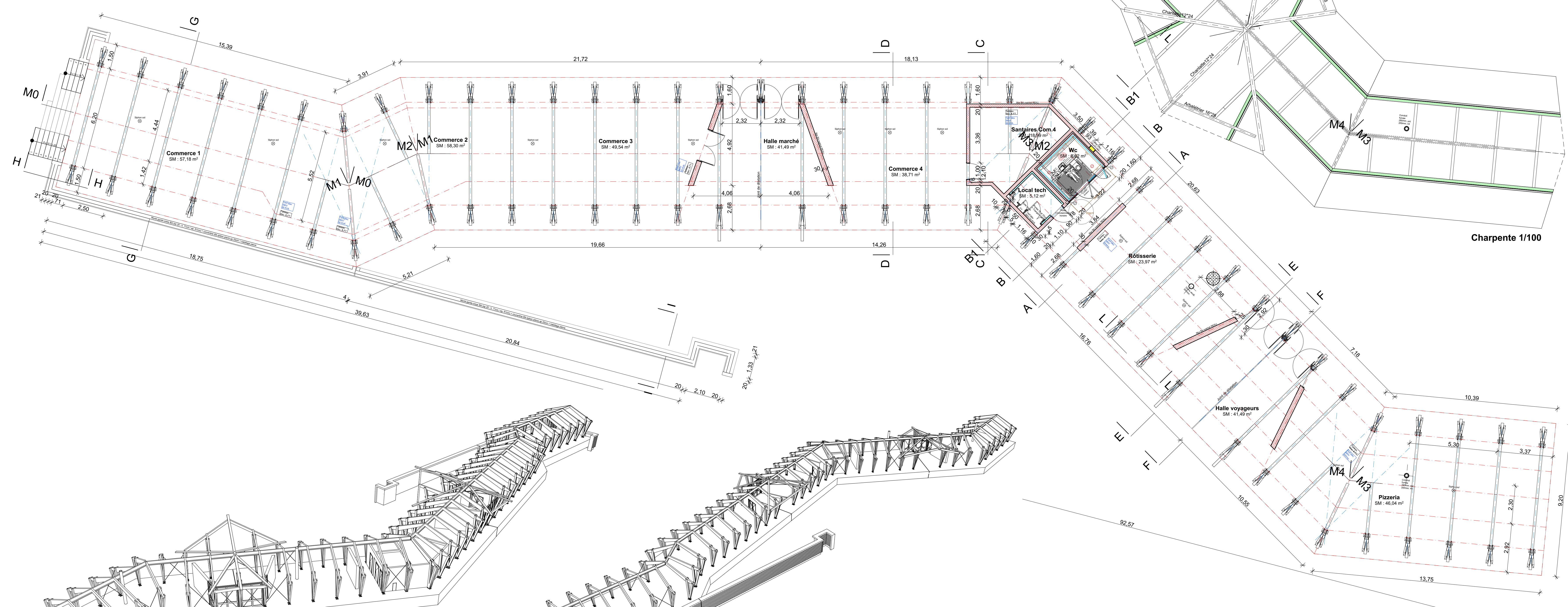
Rez de chaussée 1/100
