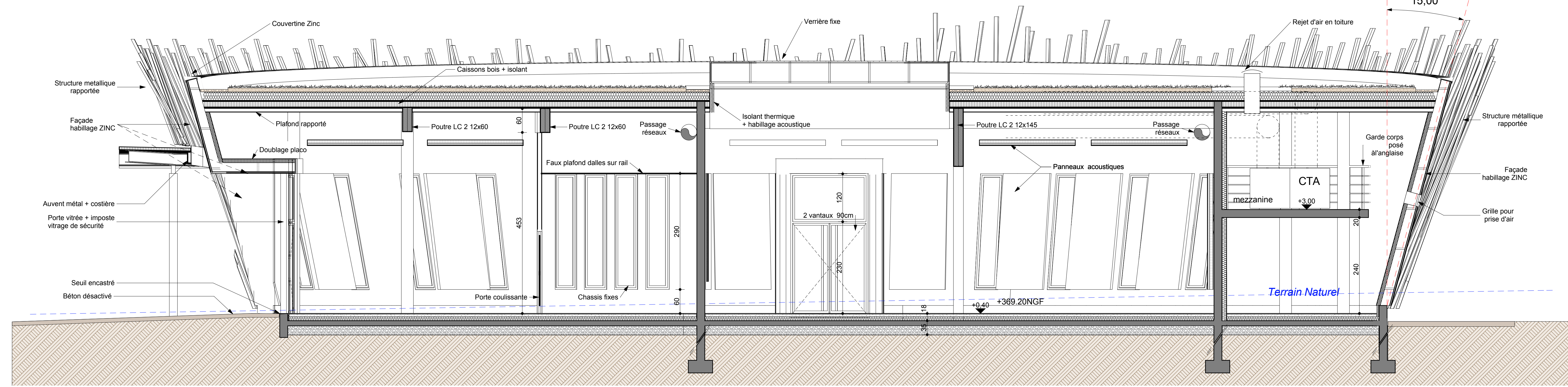
COUPE B 3
