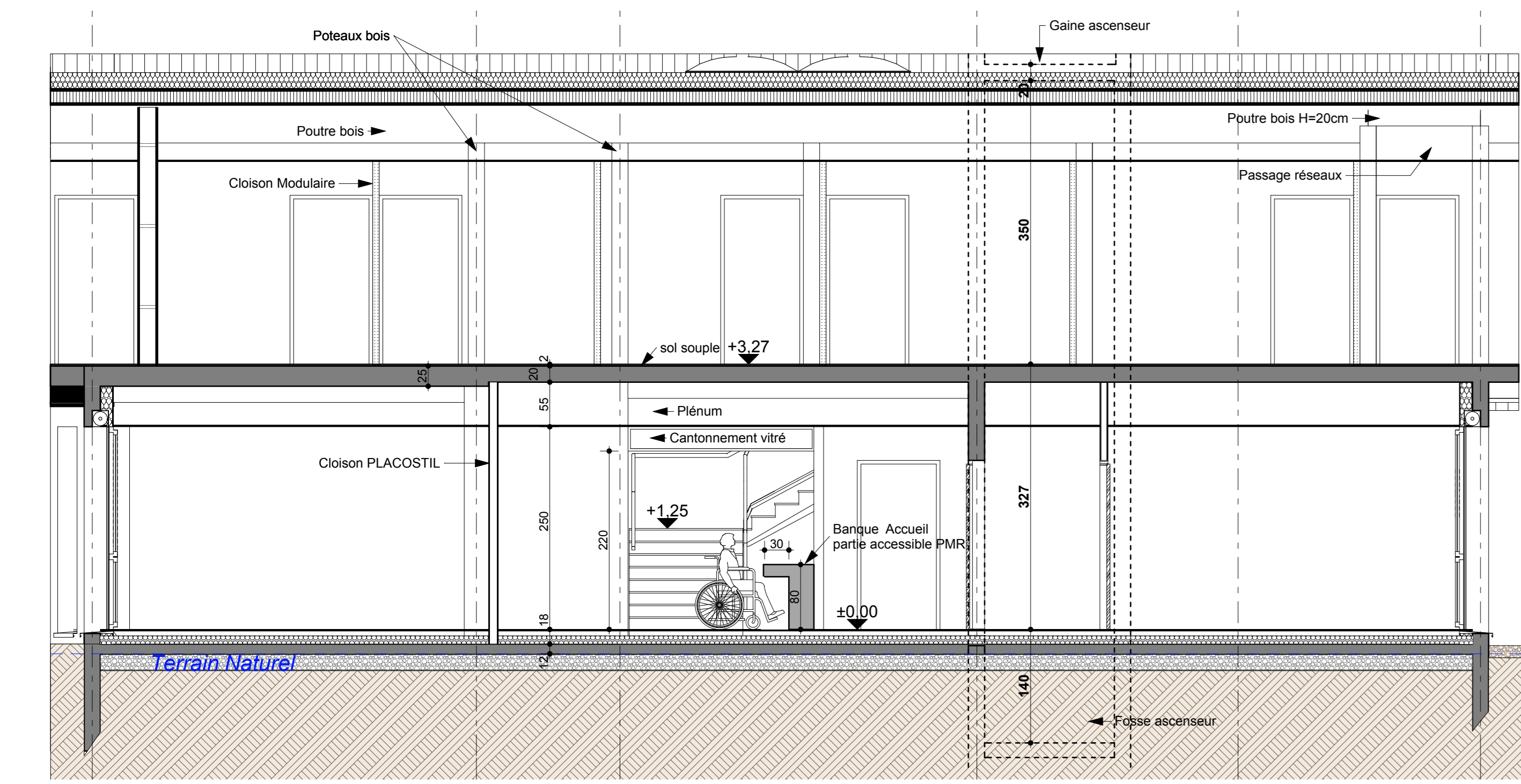
COUPE A5
