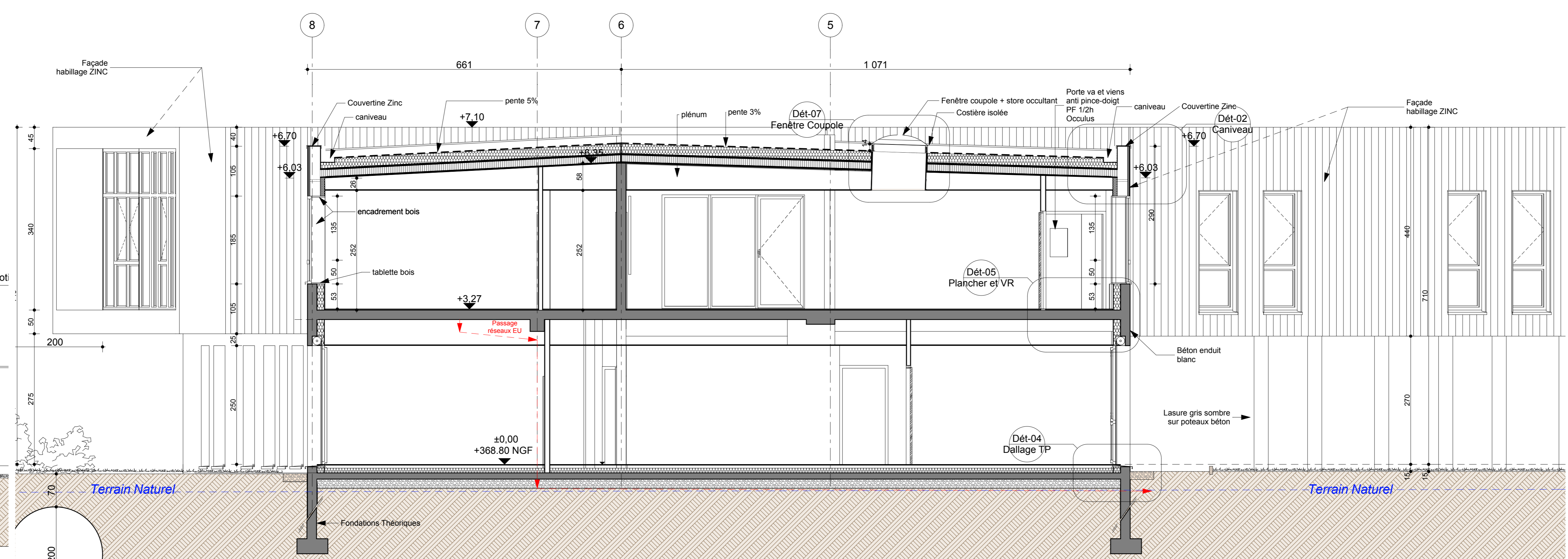
COUPE A2
