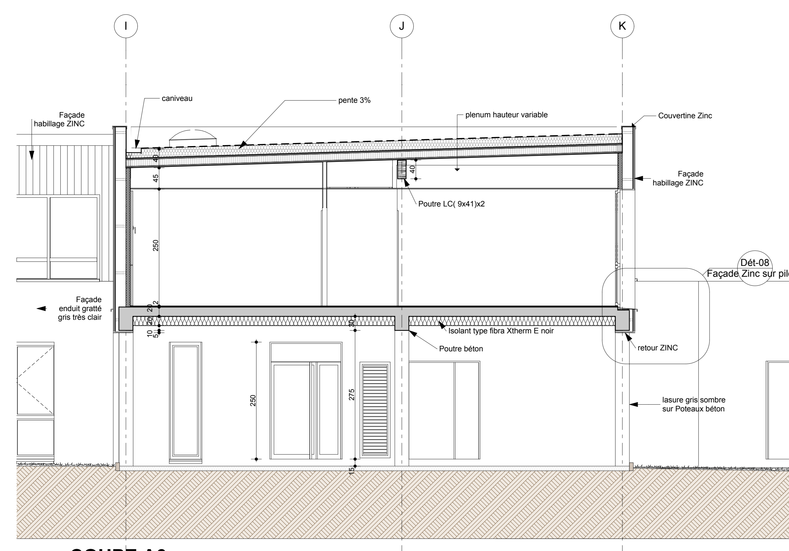
COUPE A6
