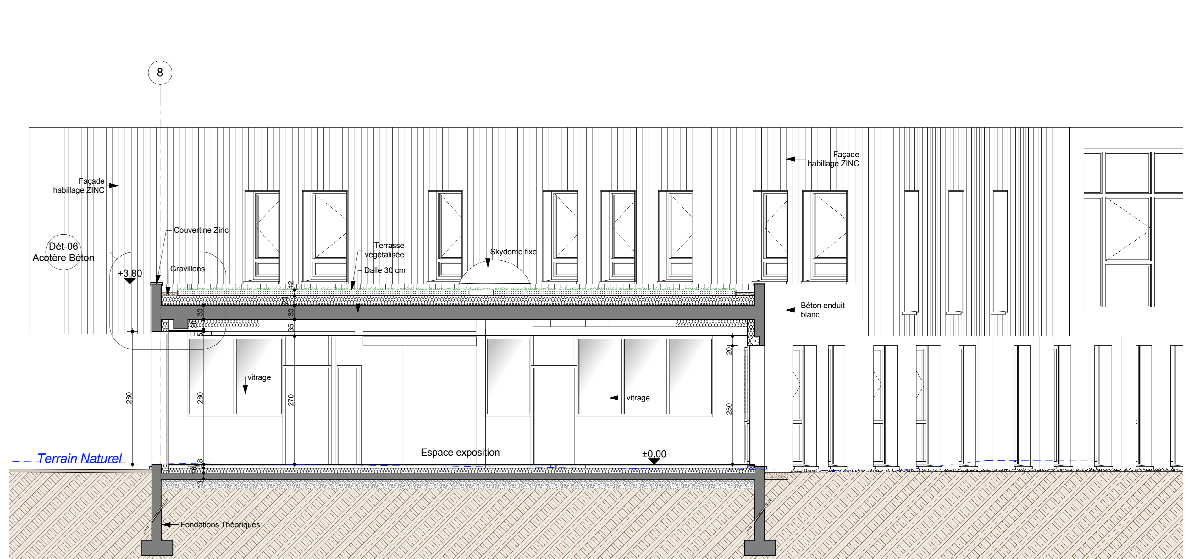
COUPE A3
