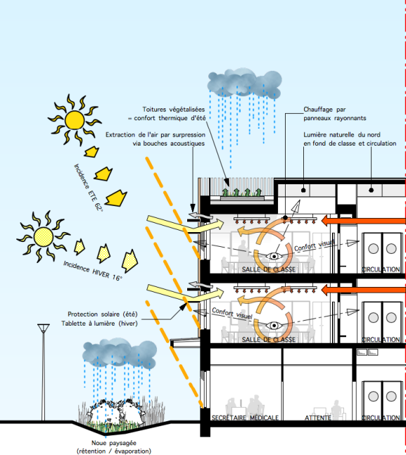
COUPE TRANSVERSALE (façade OUEST)
