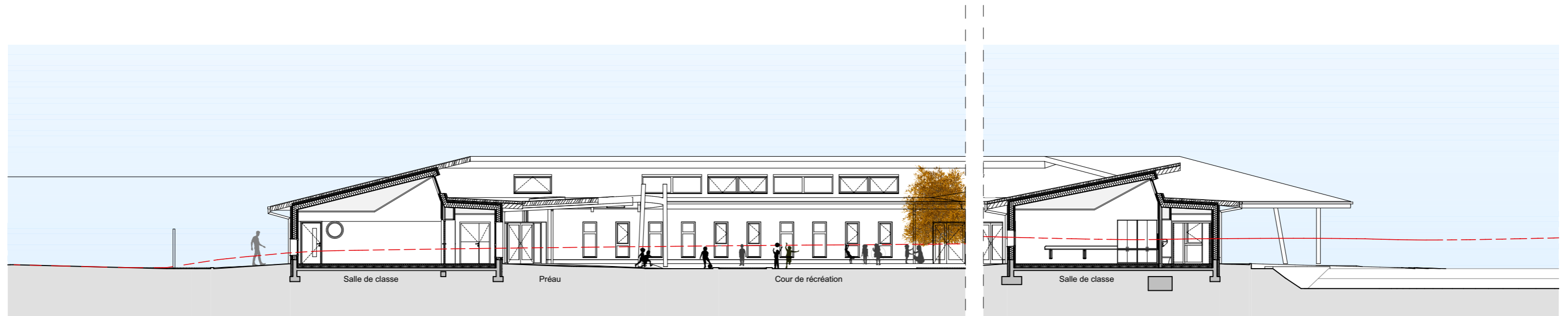
Coupe BB
