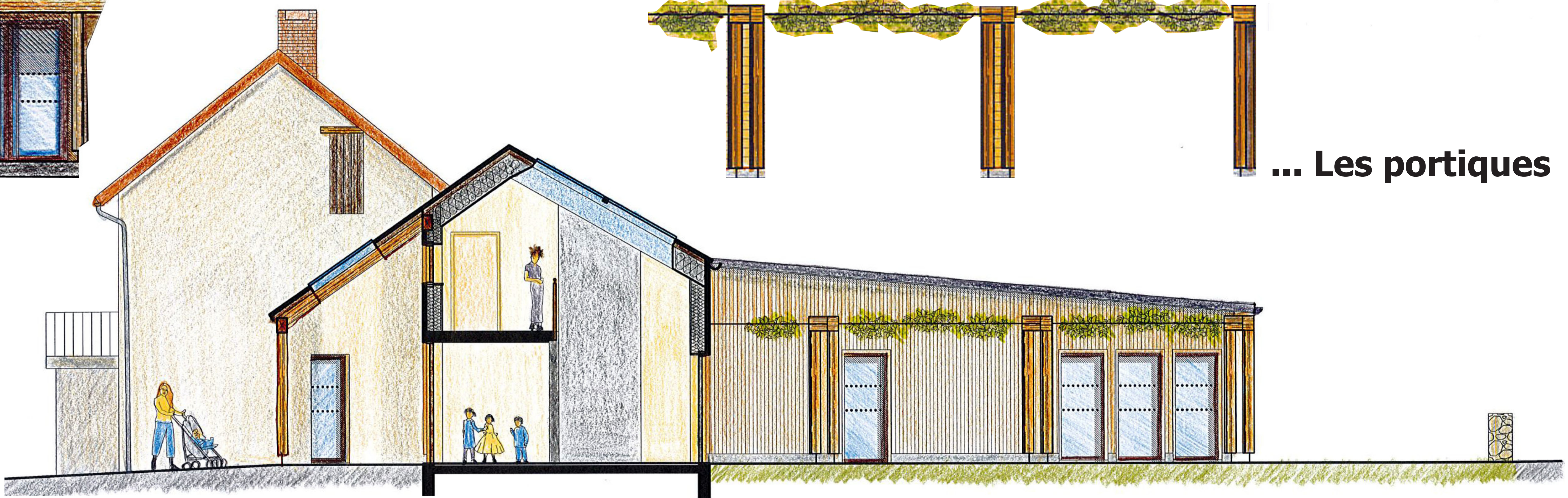
Coupe Elévation sur passage et hall d'accueil - Orientation SUD
