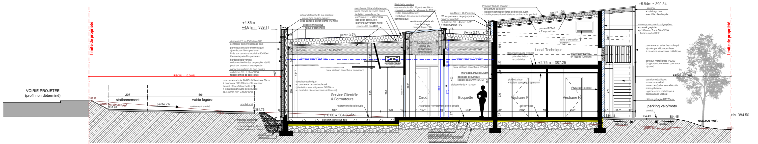
- Coupe transversale A3 sur Local Technique -
