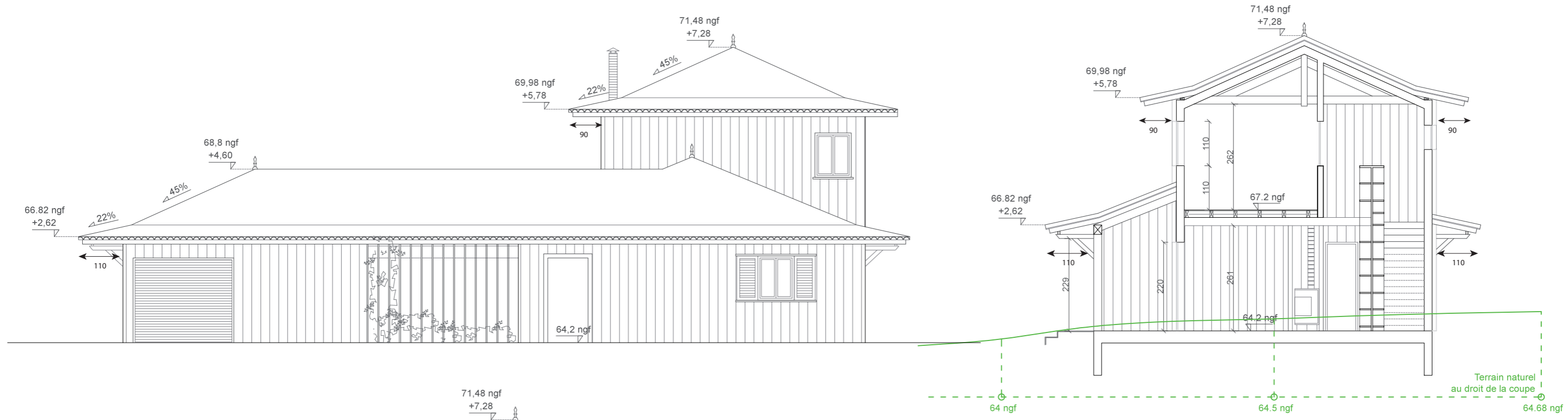
Section AA Longueur des avant-toits > 50cm
