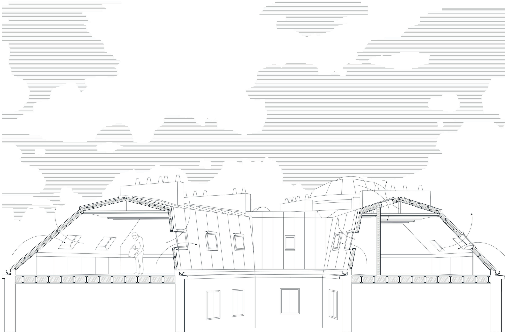
Coupe perspective
