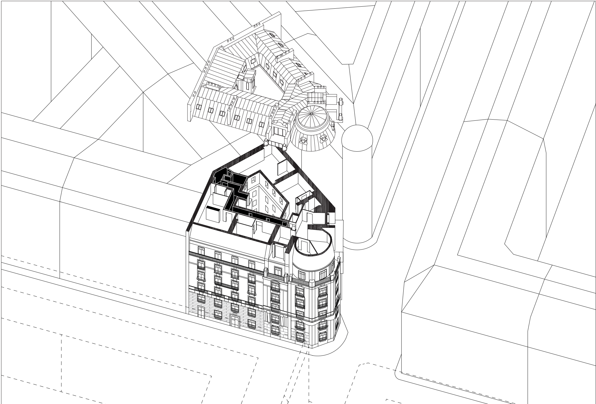
Axonometrie perspective
