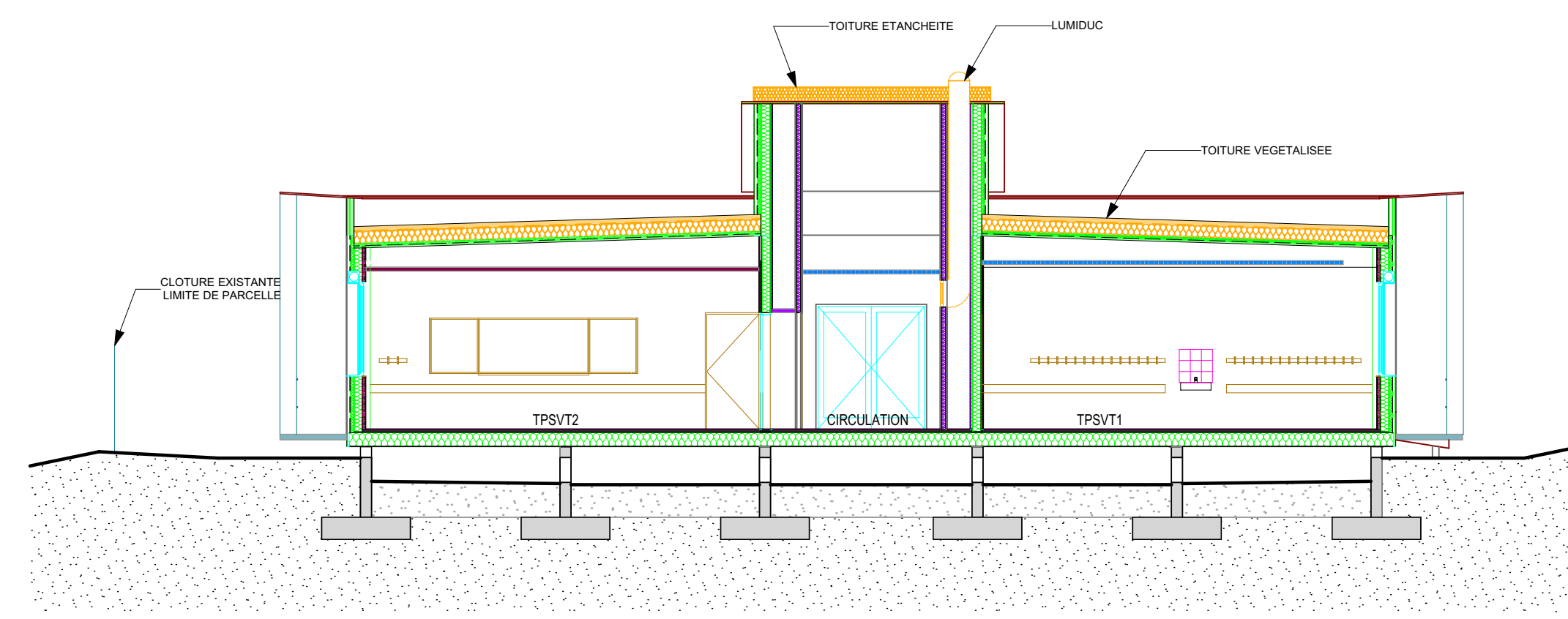
COUPE TRANSVERSALE AA
