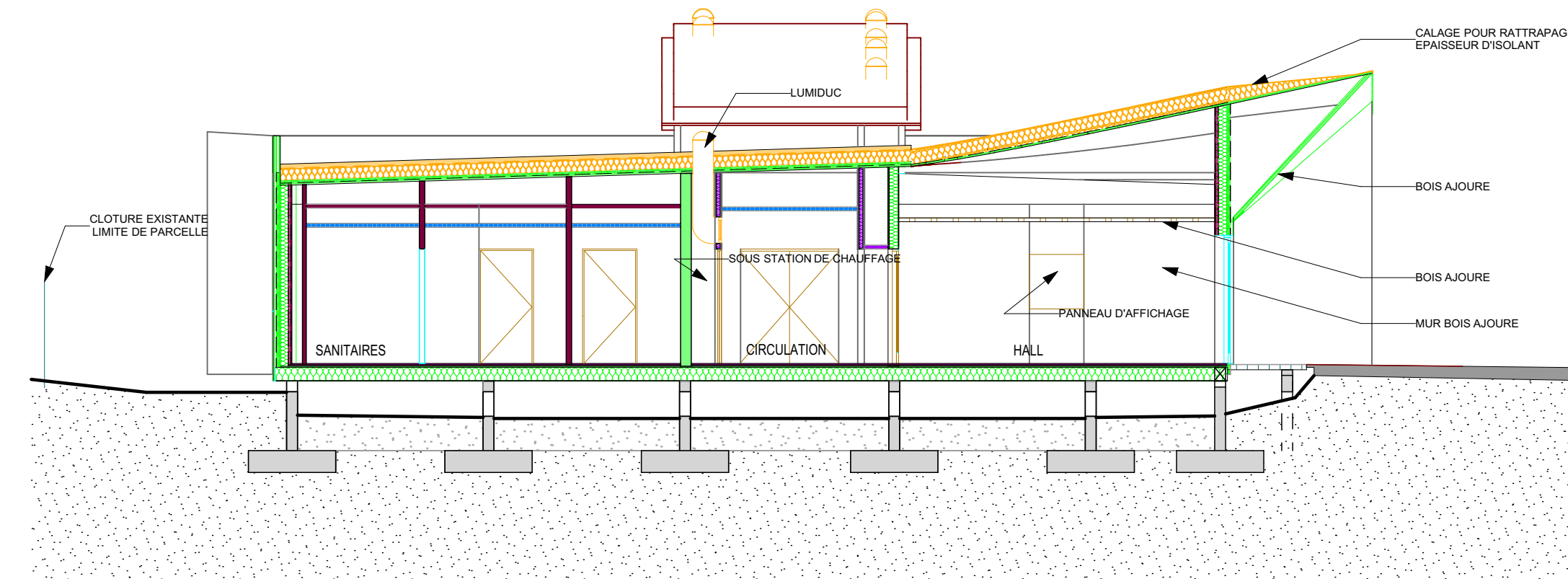
COUPE TRANSVERSALE BB
