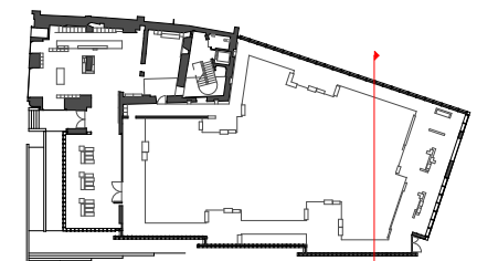
Coupe 1/200
