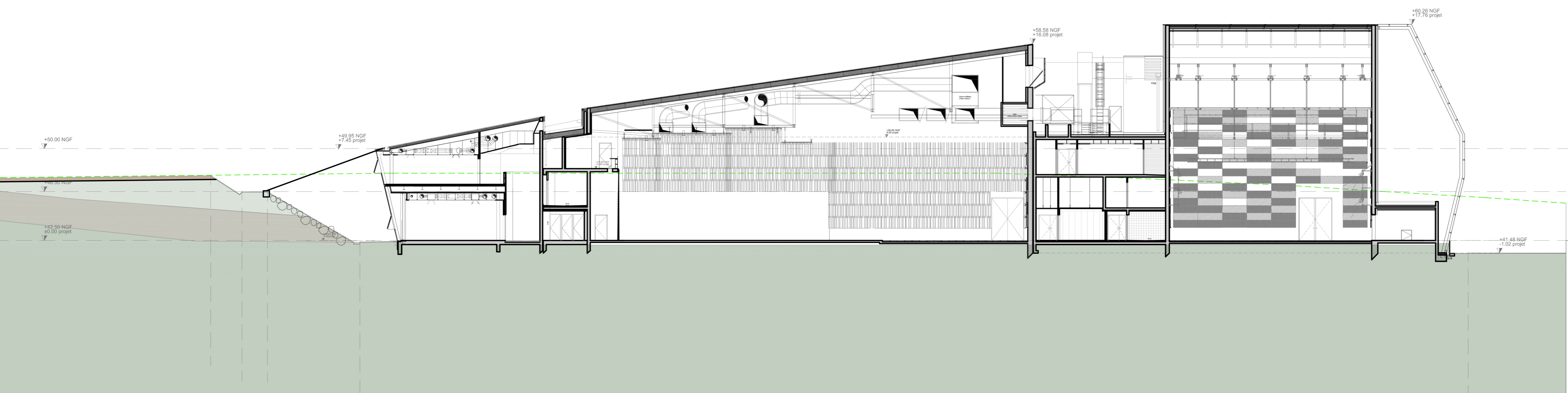
Coupe 1 : longitudinale sur l'ensemble du bâtiment et du terrain
