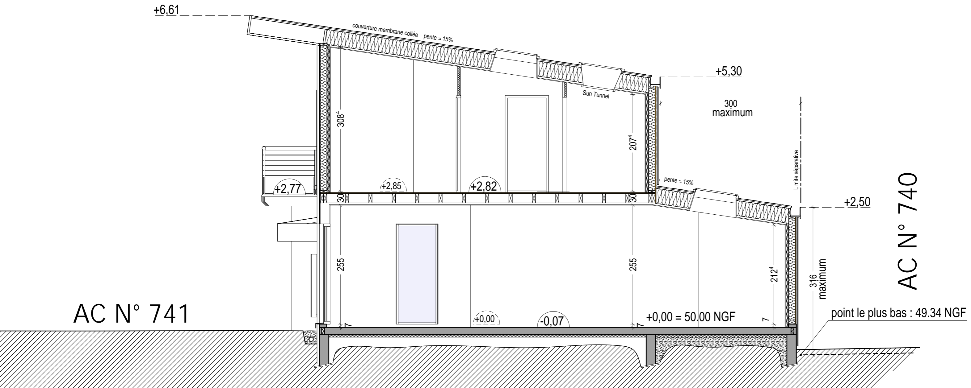
Coupe B échelle 1/50ème
