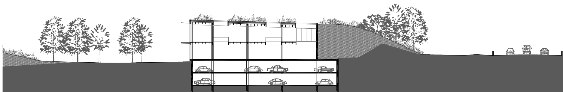
Coupe transversale
