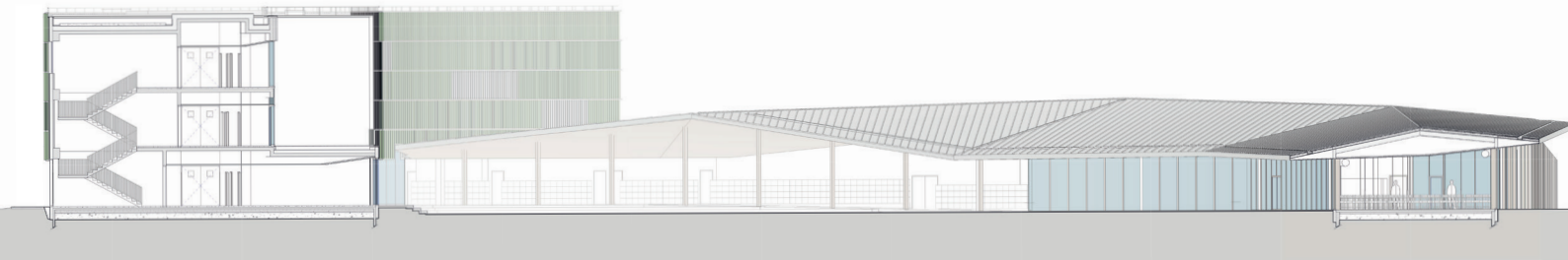
22 - Coupe collège et demi-pension
