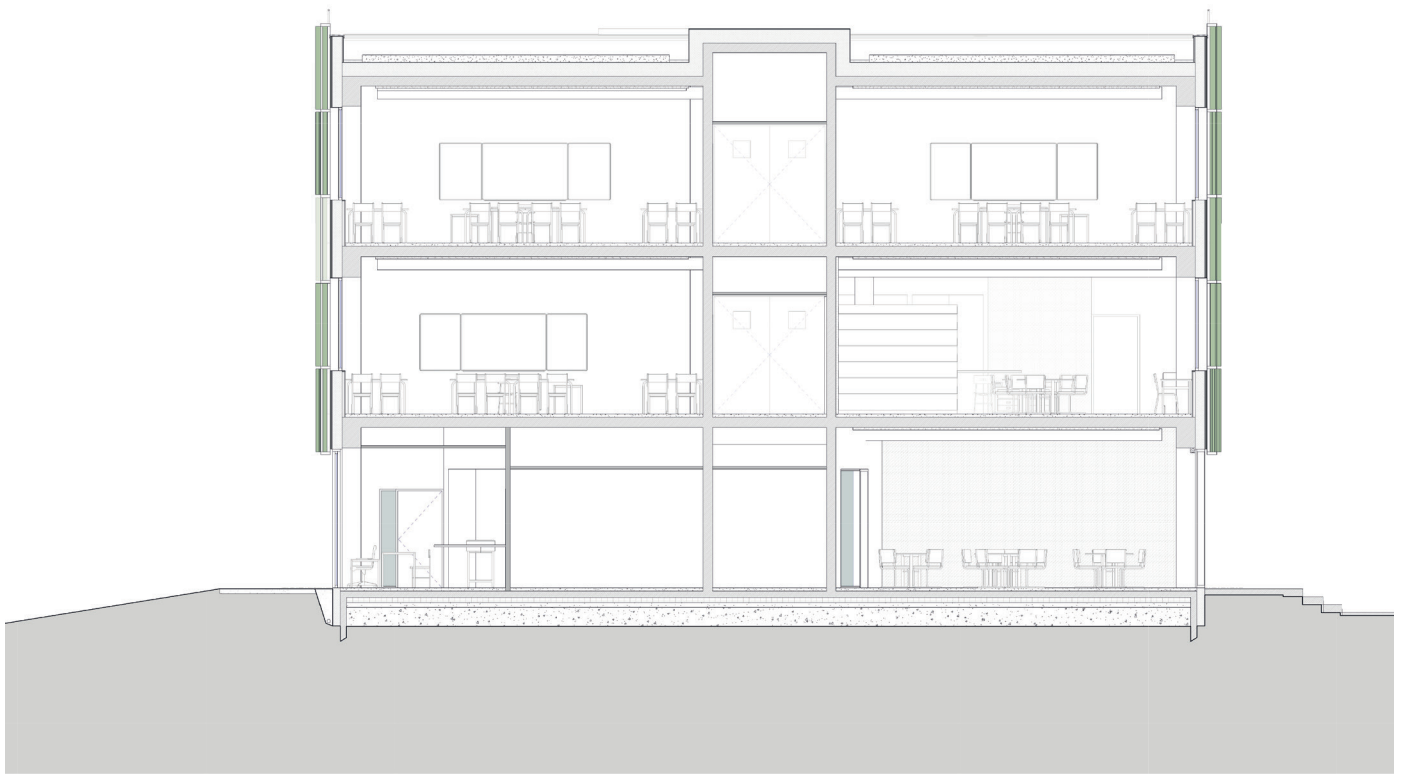
21 - Coupe transversale collège
