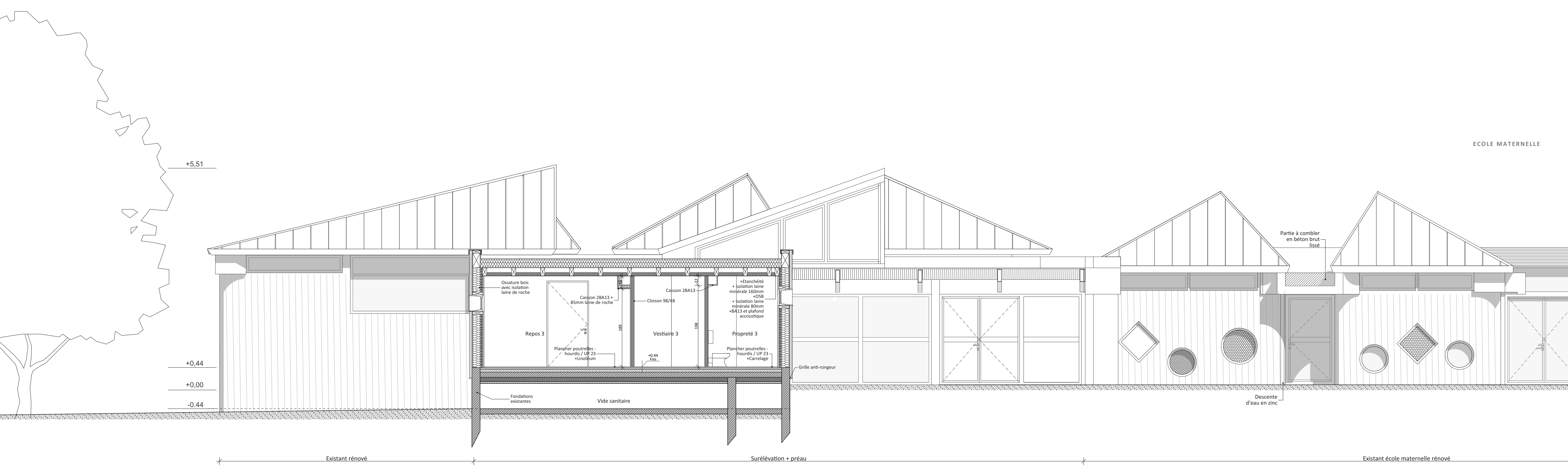
Coupe A-A
