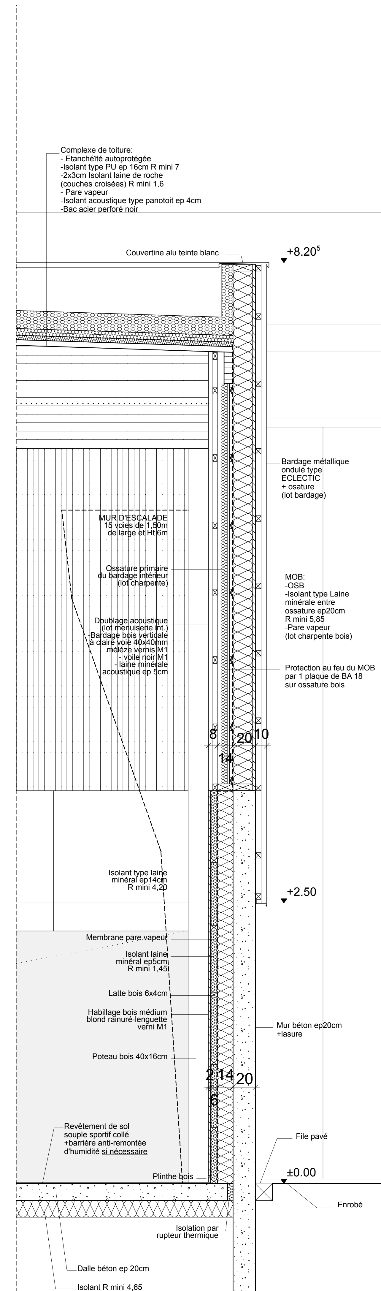
COUPE DETAIL 2 FACADE OUEST EXTENSION
