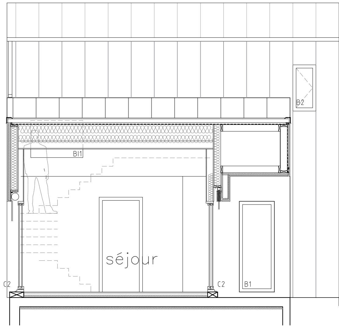
Coupe BB
