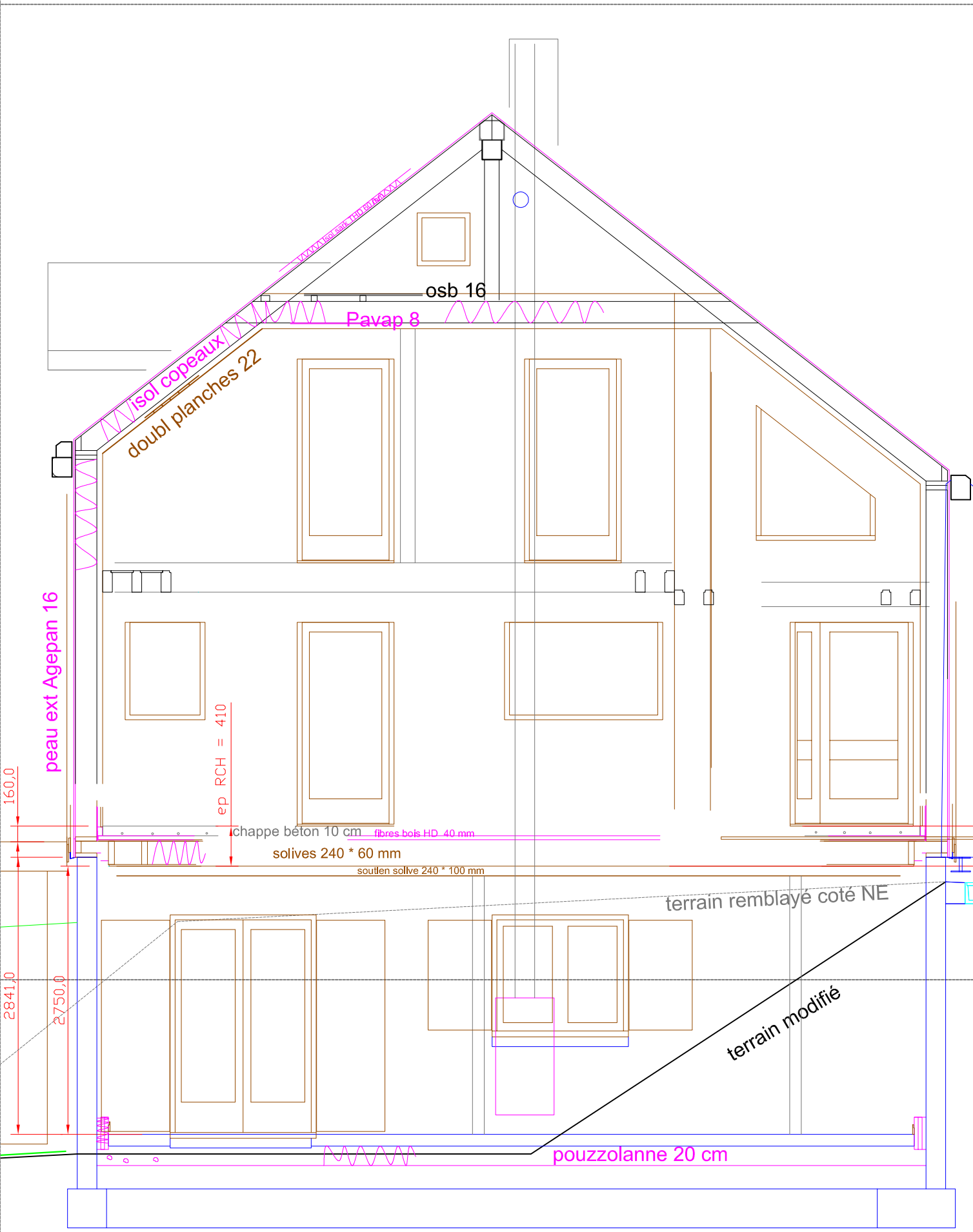
Coupe et vue int et isol SW 13 mars 11
