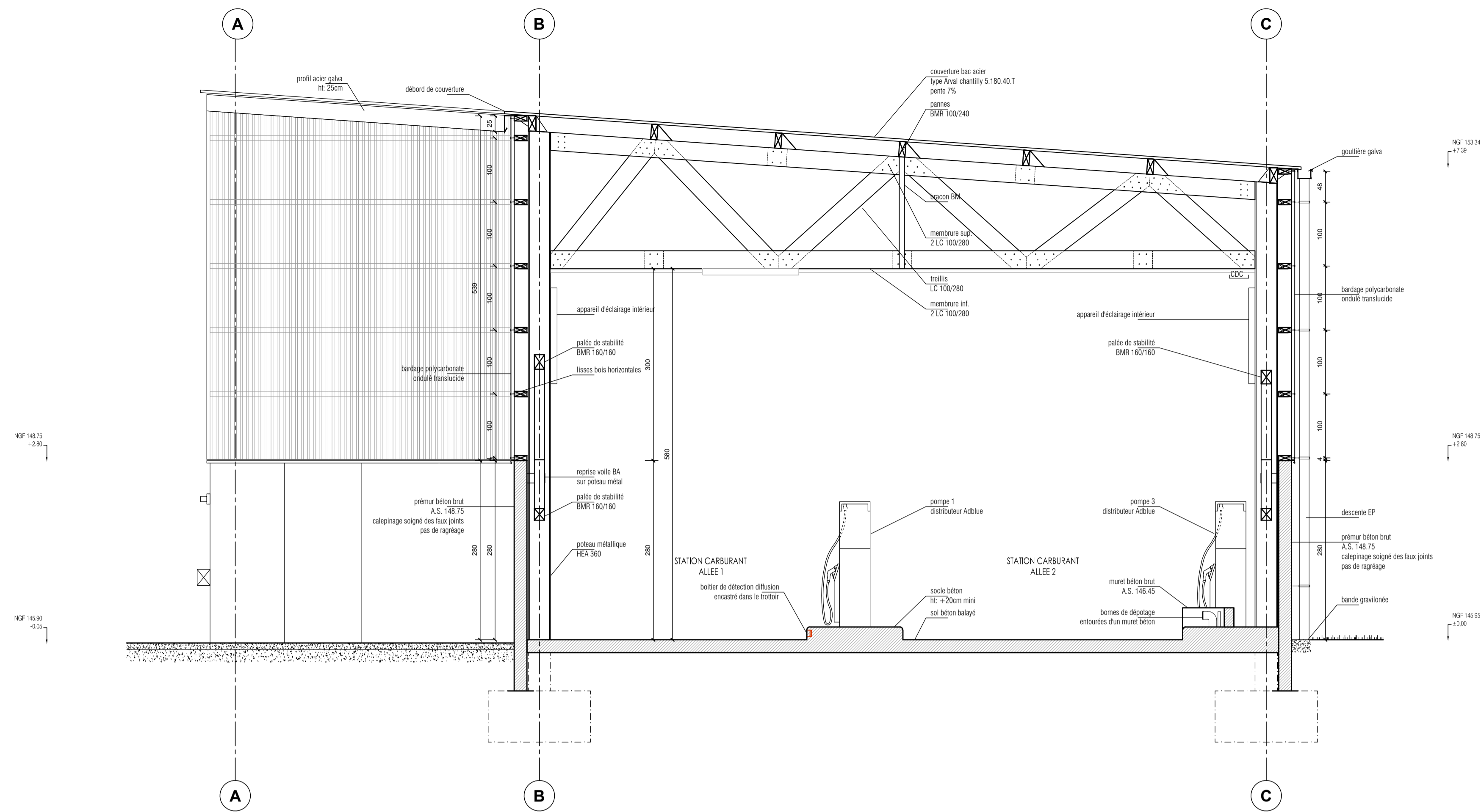
BATIMENT C - COUPE A - 1/50
