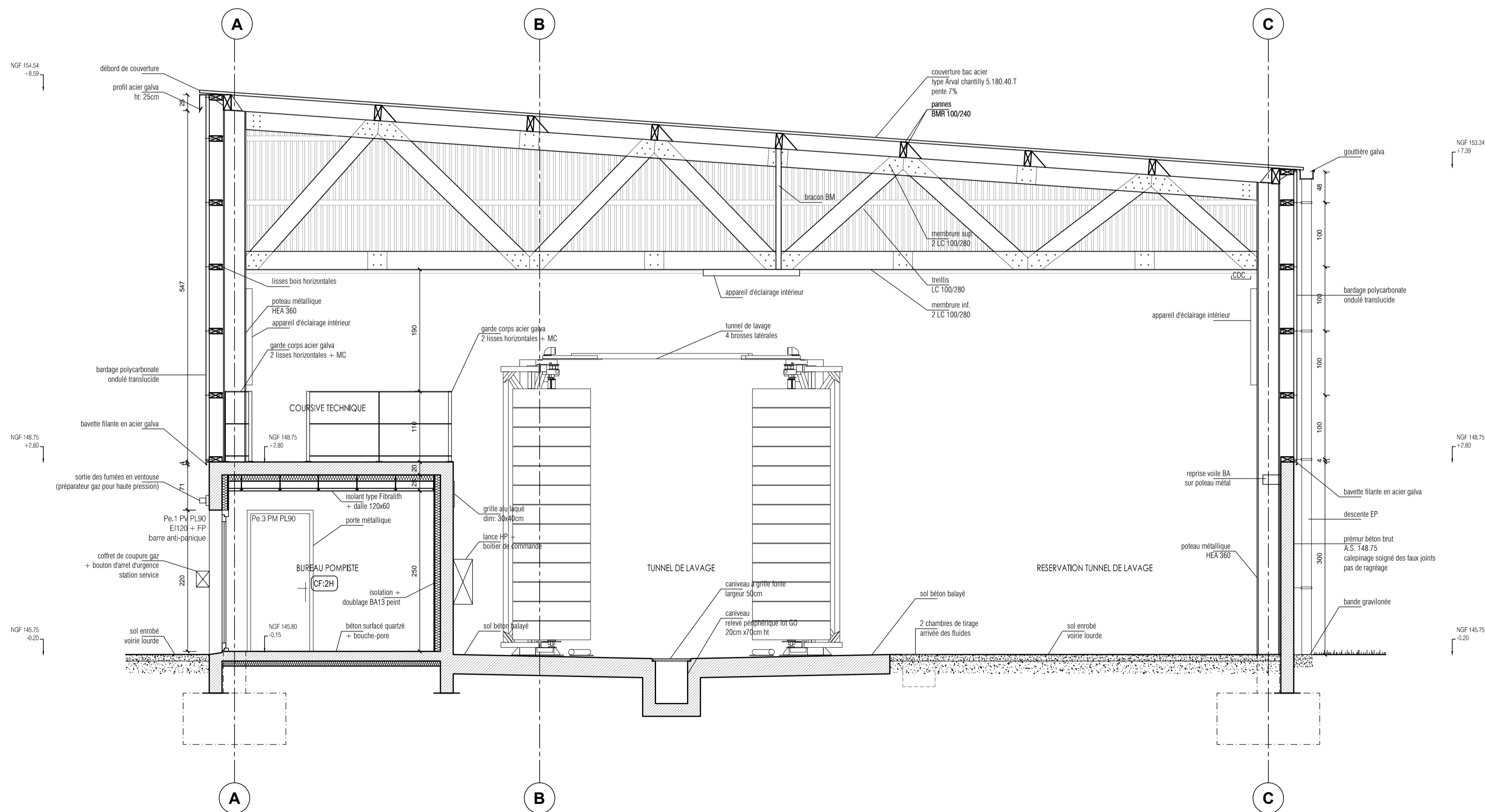
BATIMENT C - COUPE B - 1/50
