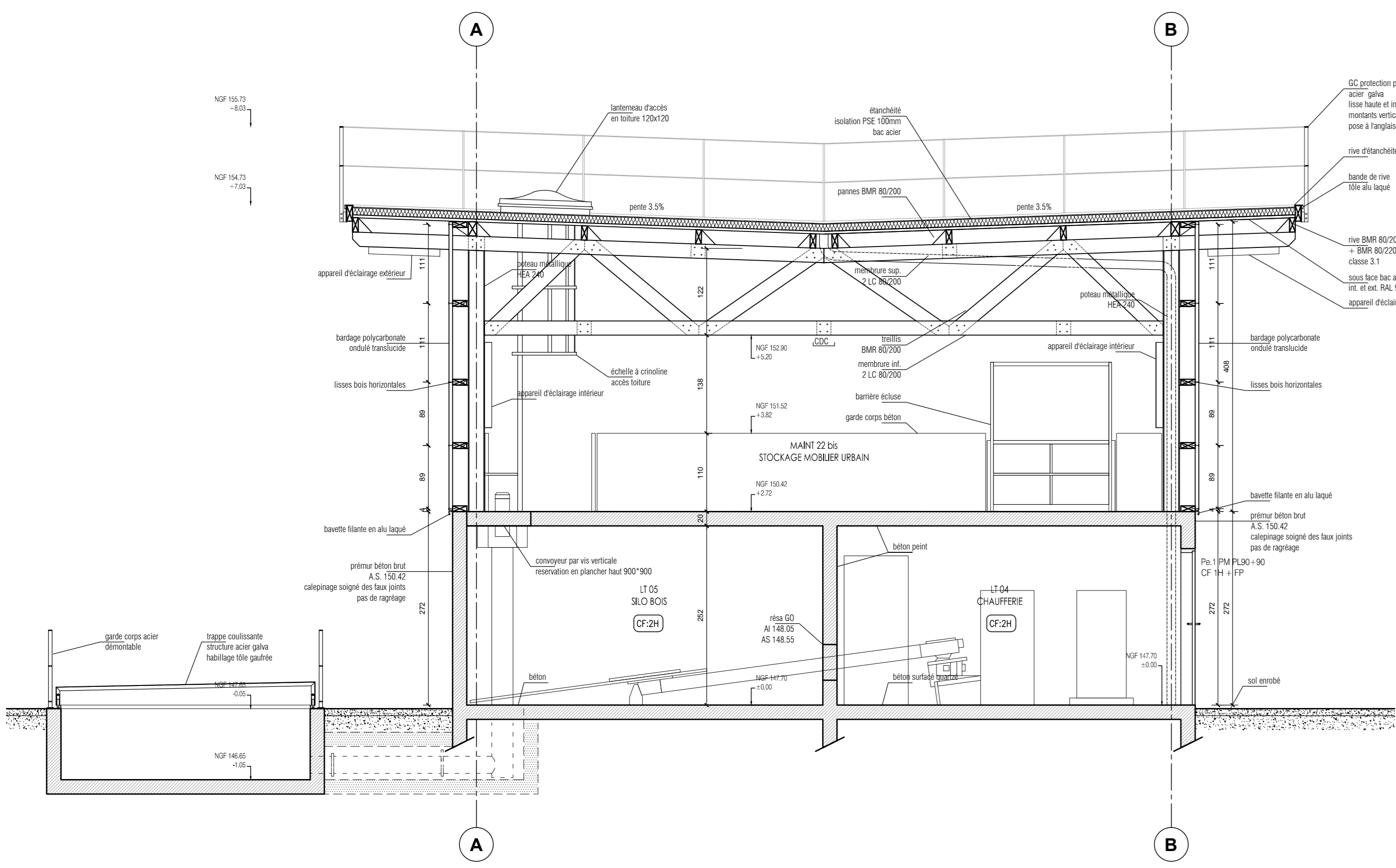
BATIMENT B - COUPE A
