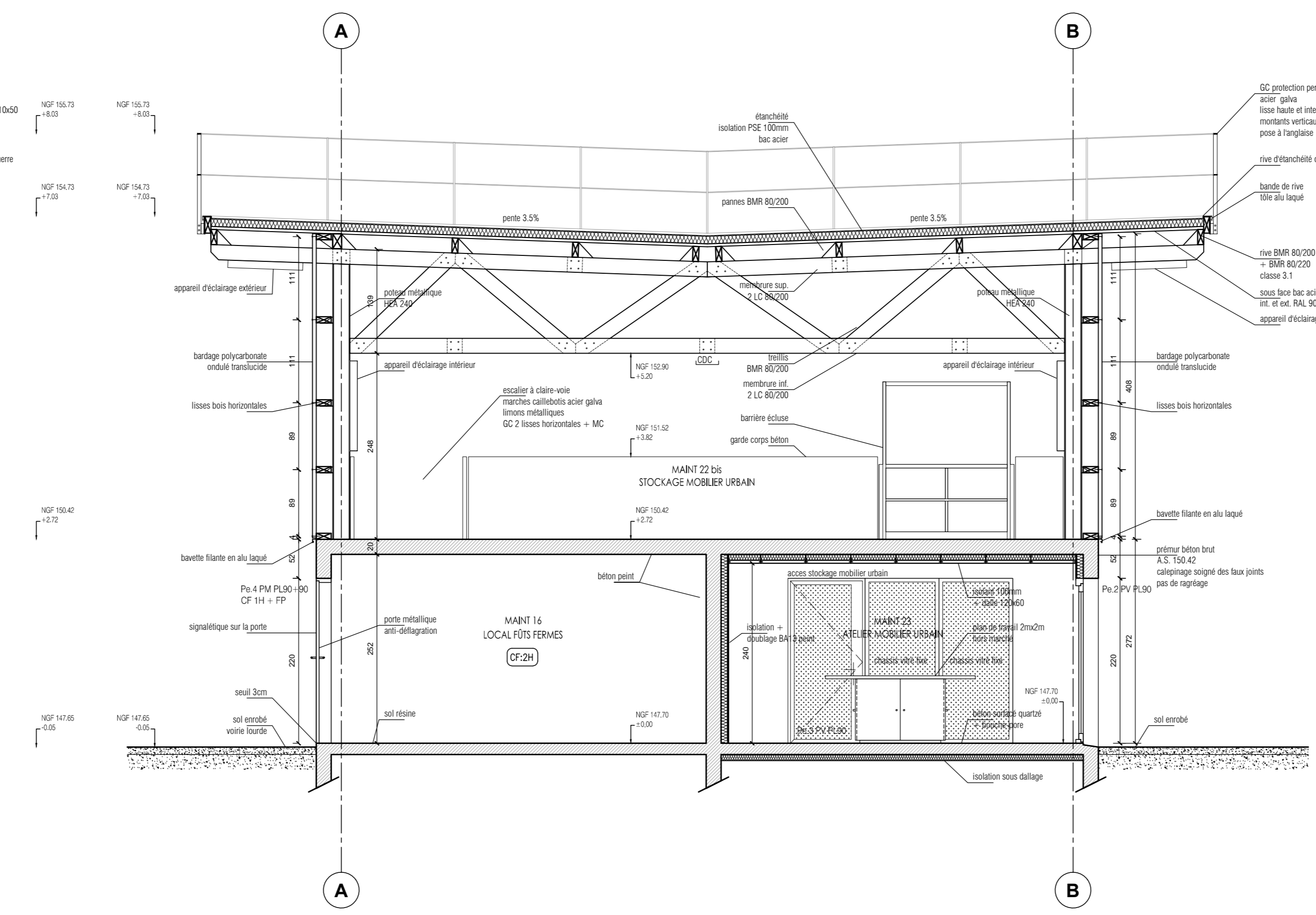
BATIMENT B - COUPE B
