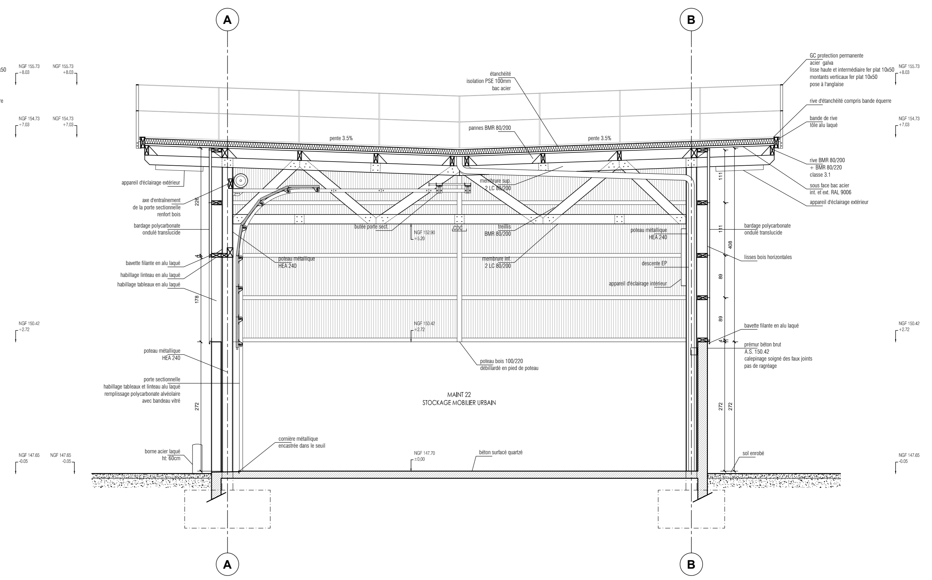
BATIMENT B - COUPE C
