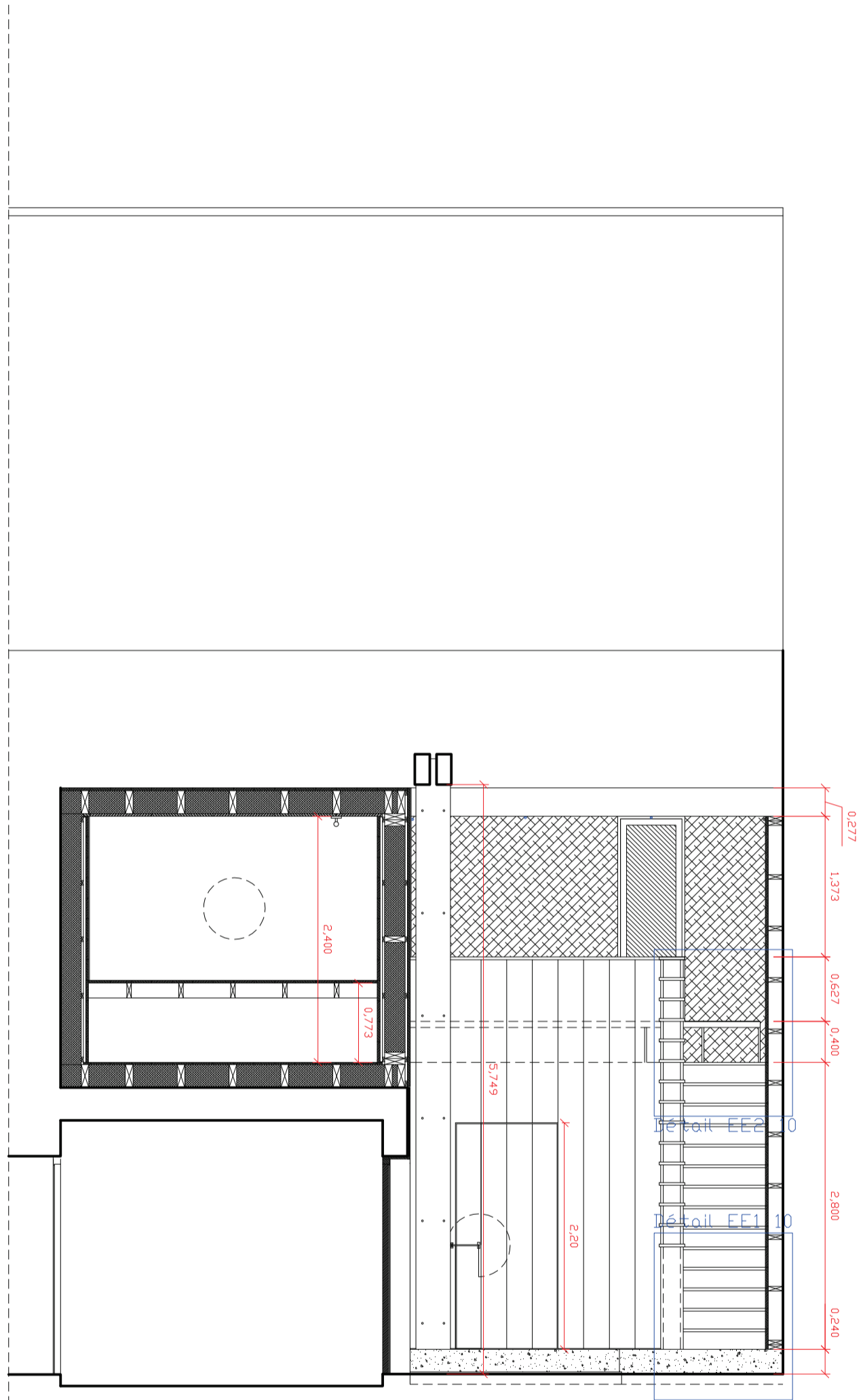
Coupe EE
