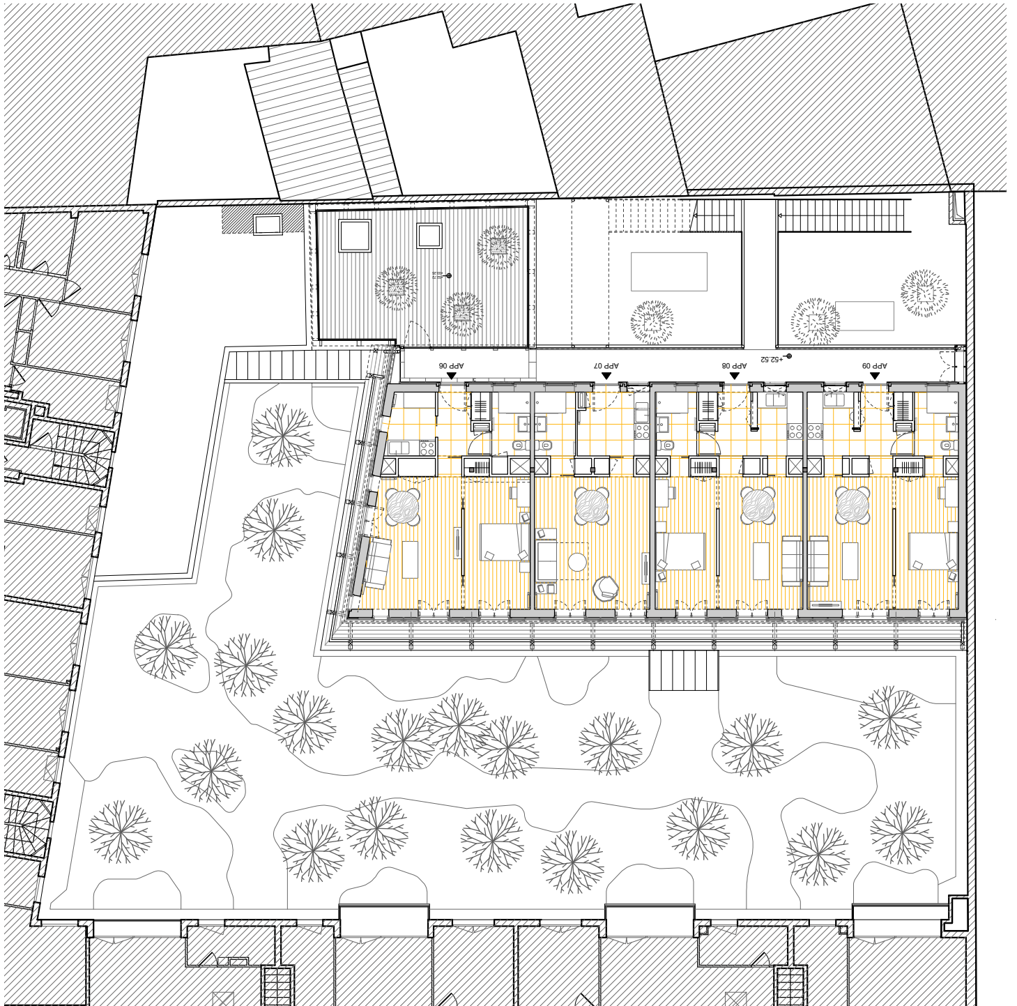
Premier étage 1/200
