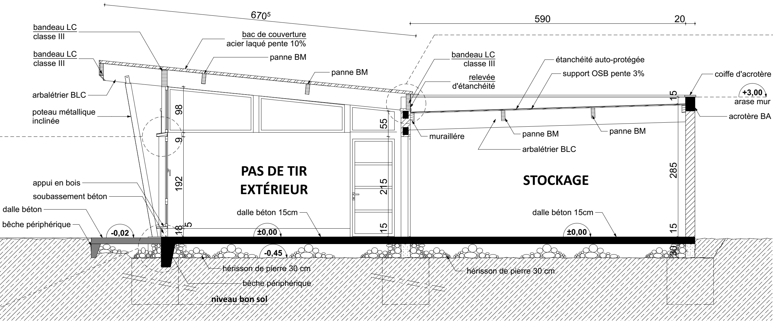
COUPE AA
