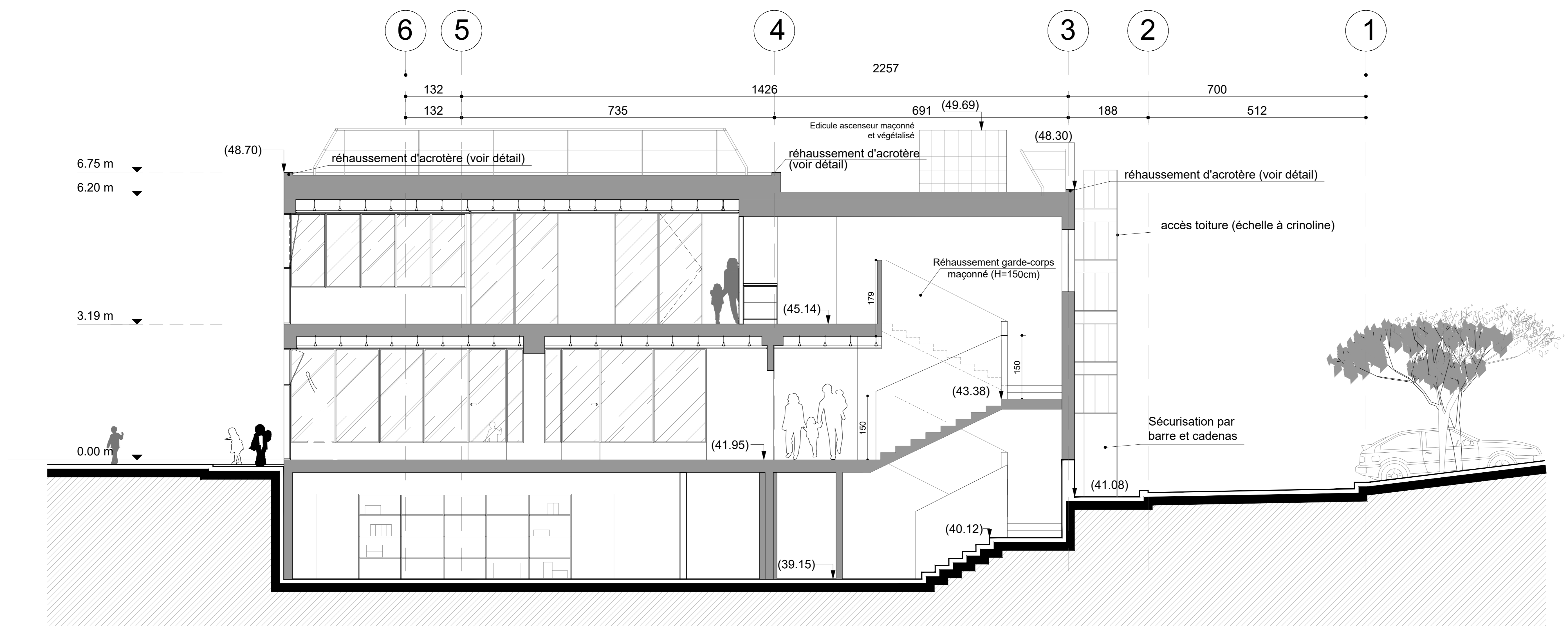
COUPE BB' - 1/50
