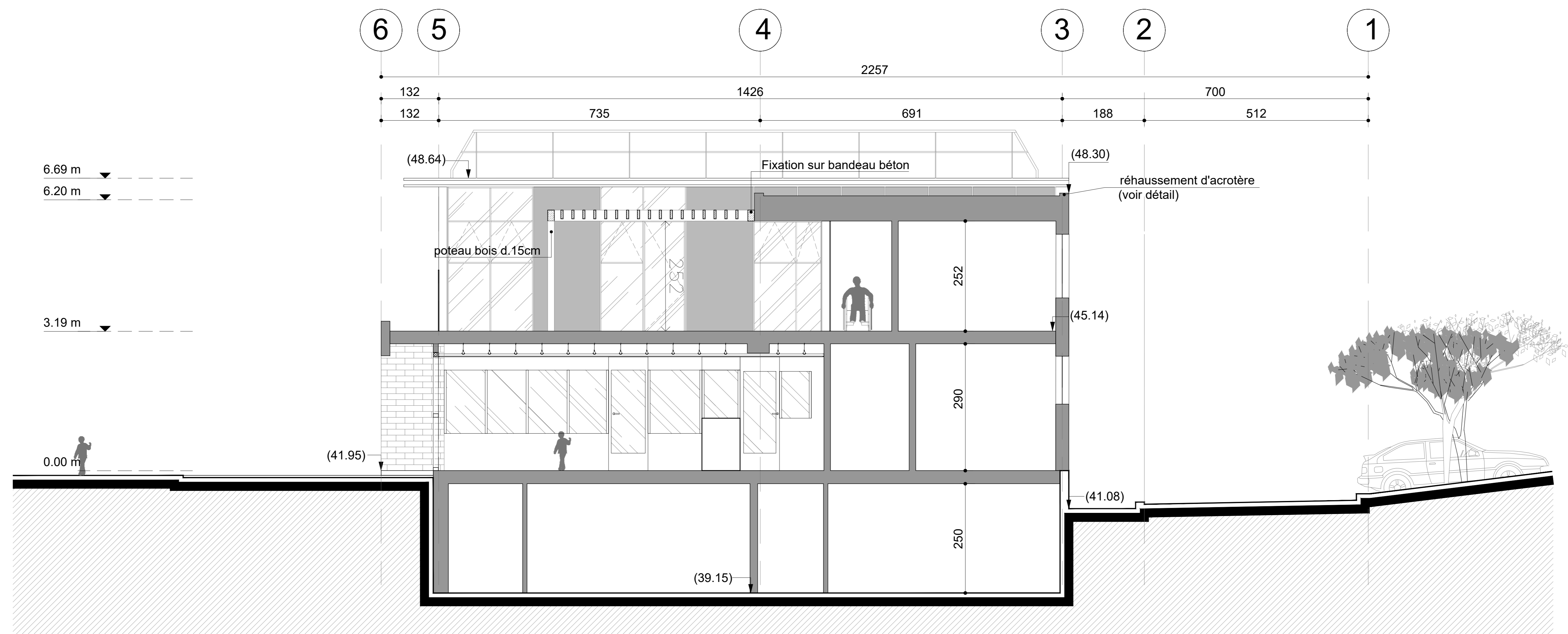
COUPE CC' - 1/50
