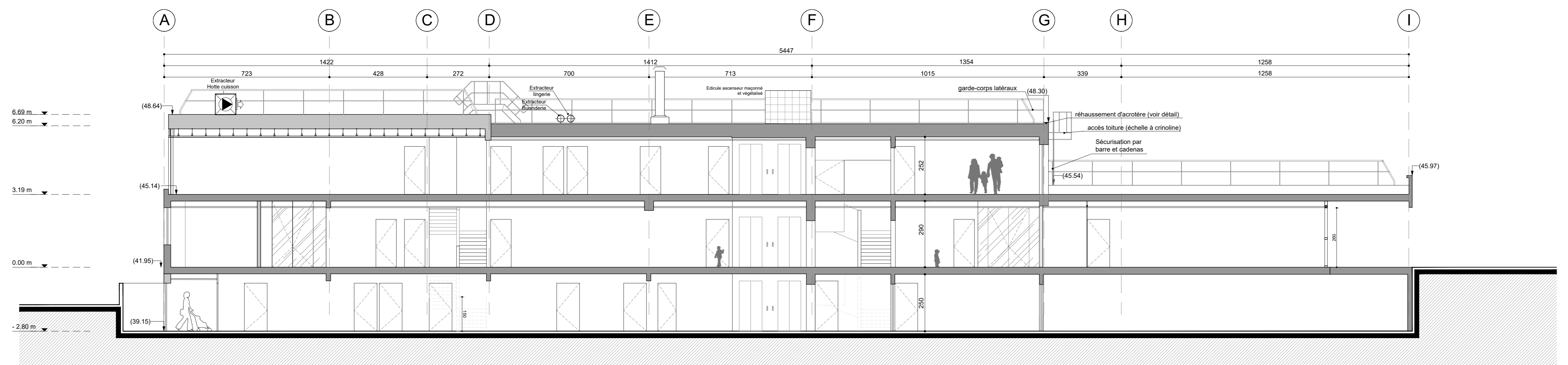
COUPE AA' - 1/100
