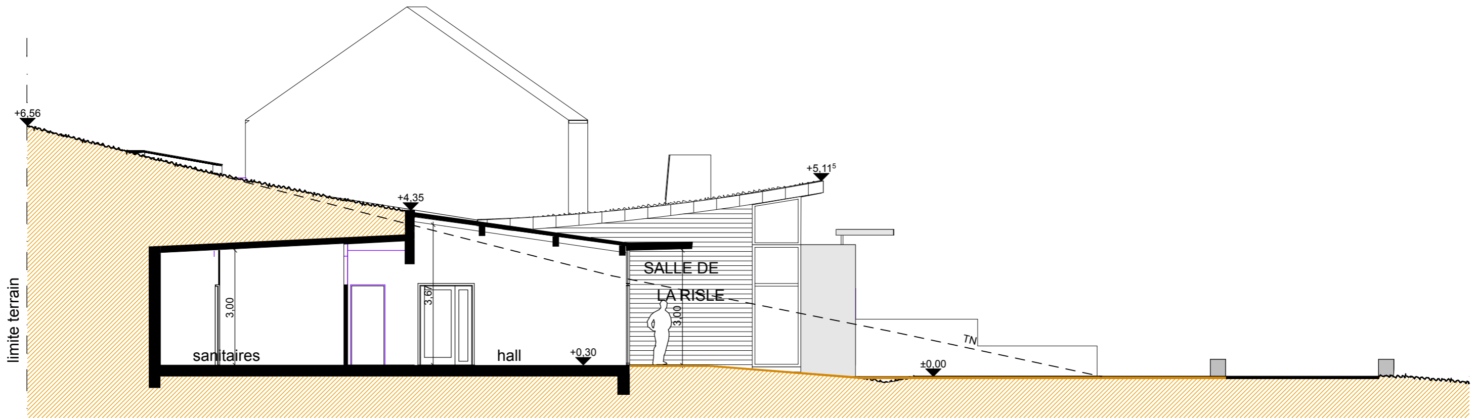
coupe D
