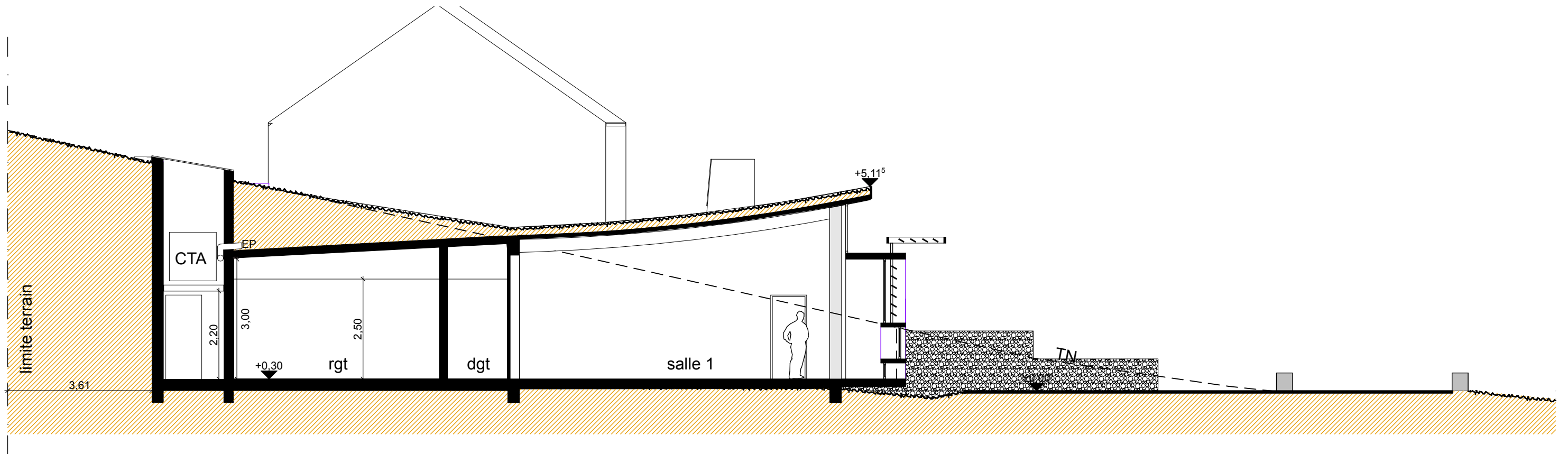
coupe A
