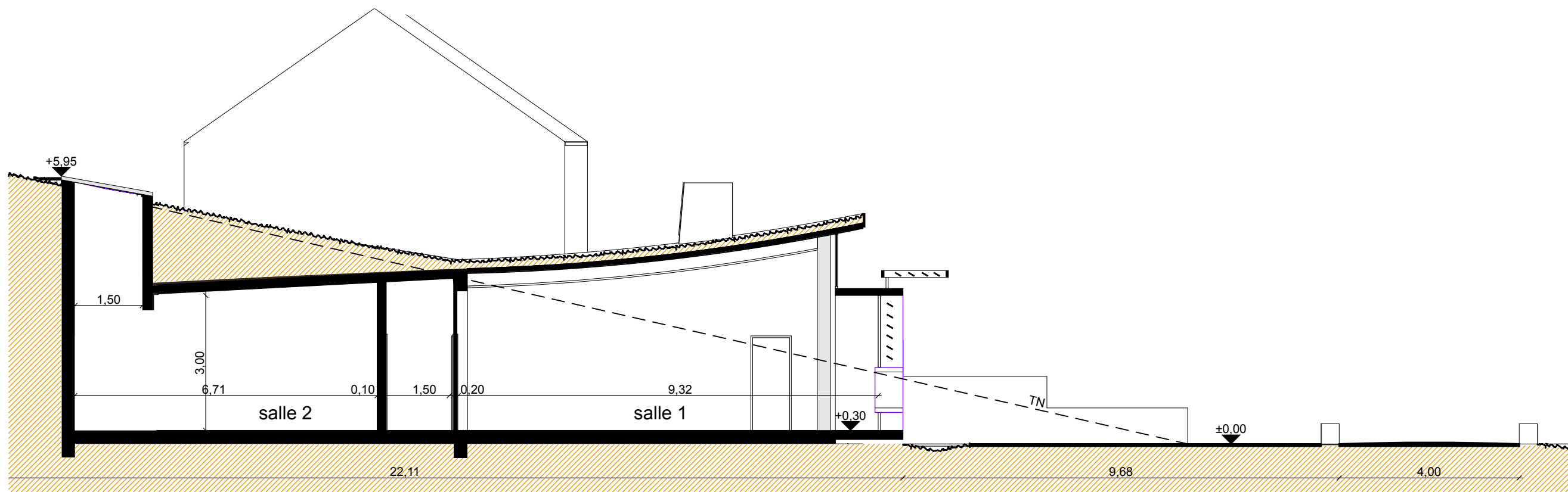
coupe B
