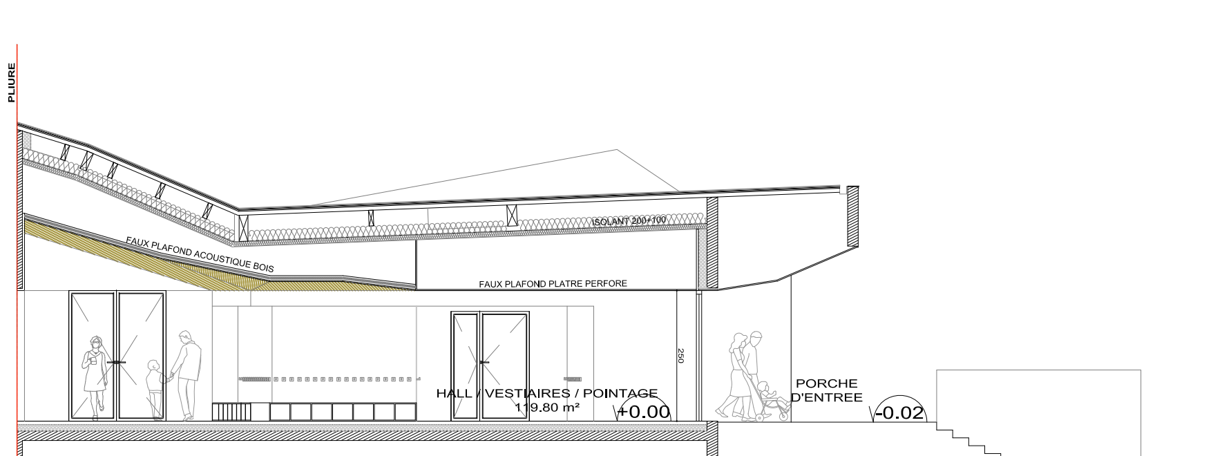
COUPE BB (partie 2)
