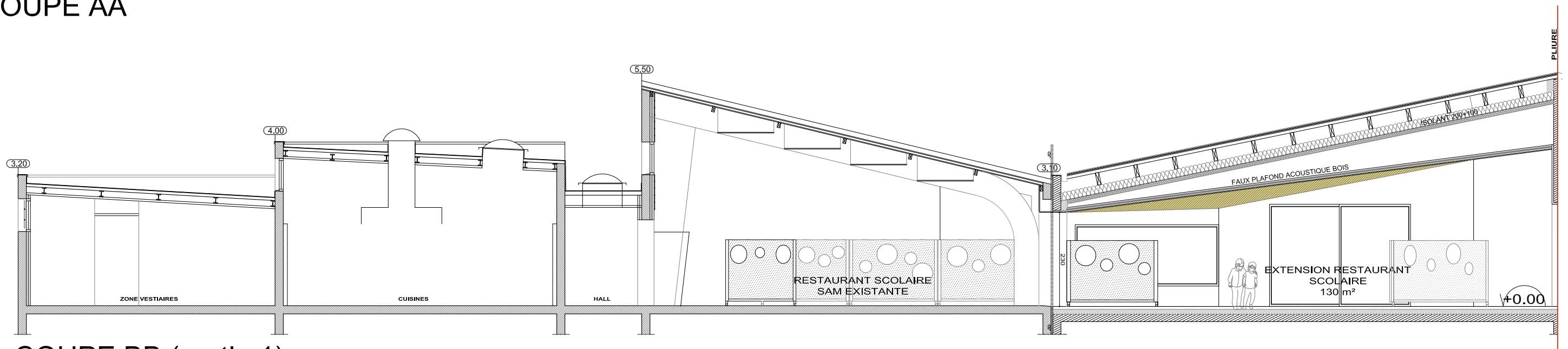
COUPE BB (partie 1)
