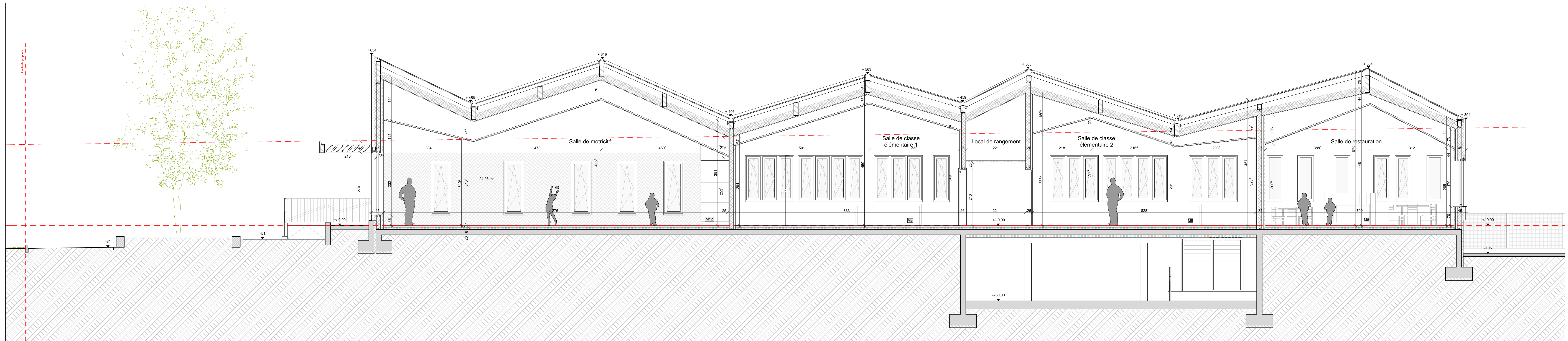
Coupe AA 1/50
