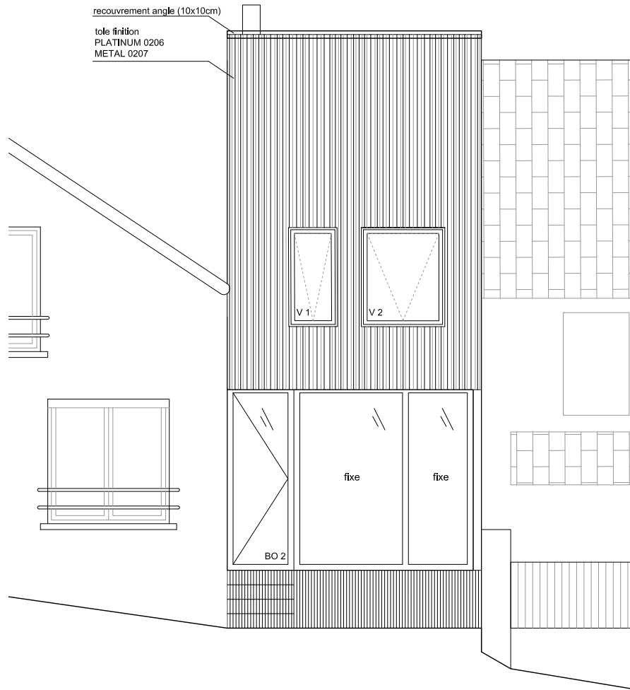
FACADE NORD
