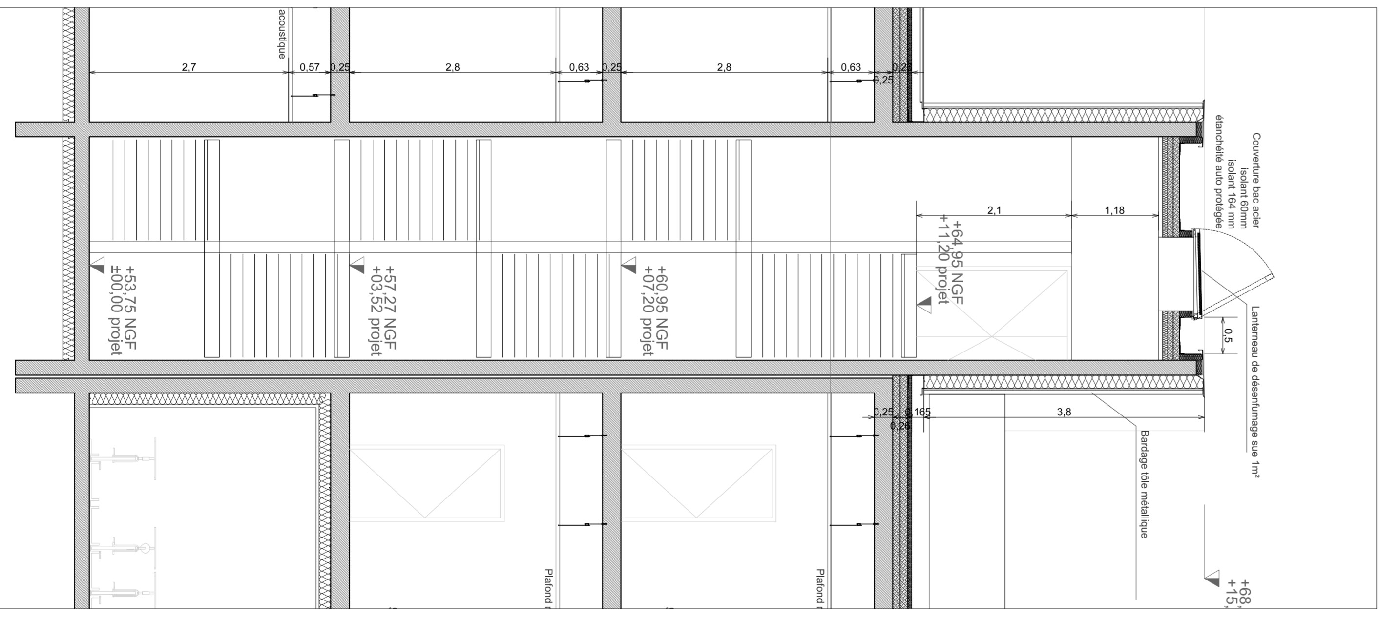
COUPE DETAIL 3 - Ech 1/50
