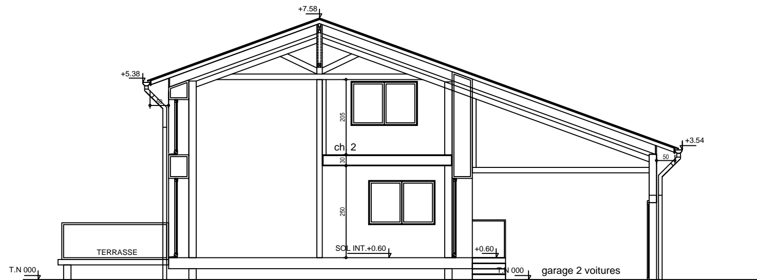
COUPE A - A
