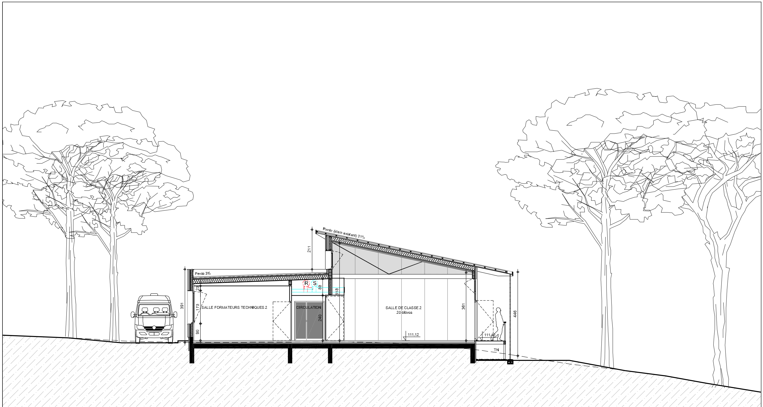
COUPE AA sur bâtiment d'enseignement - 1/100
