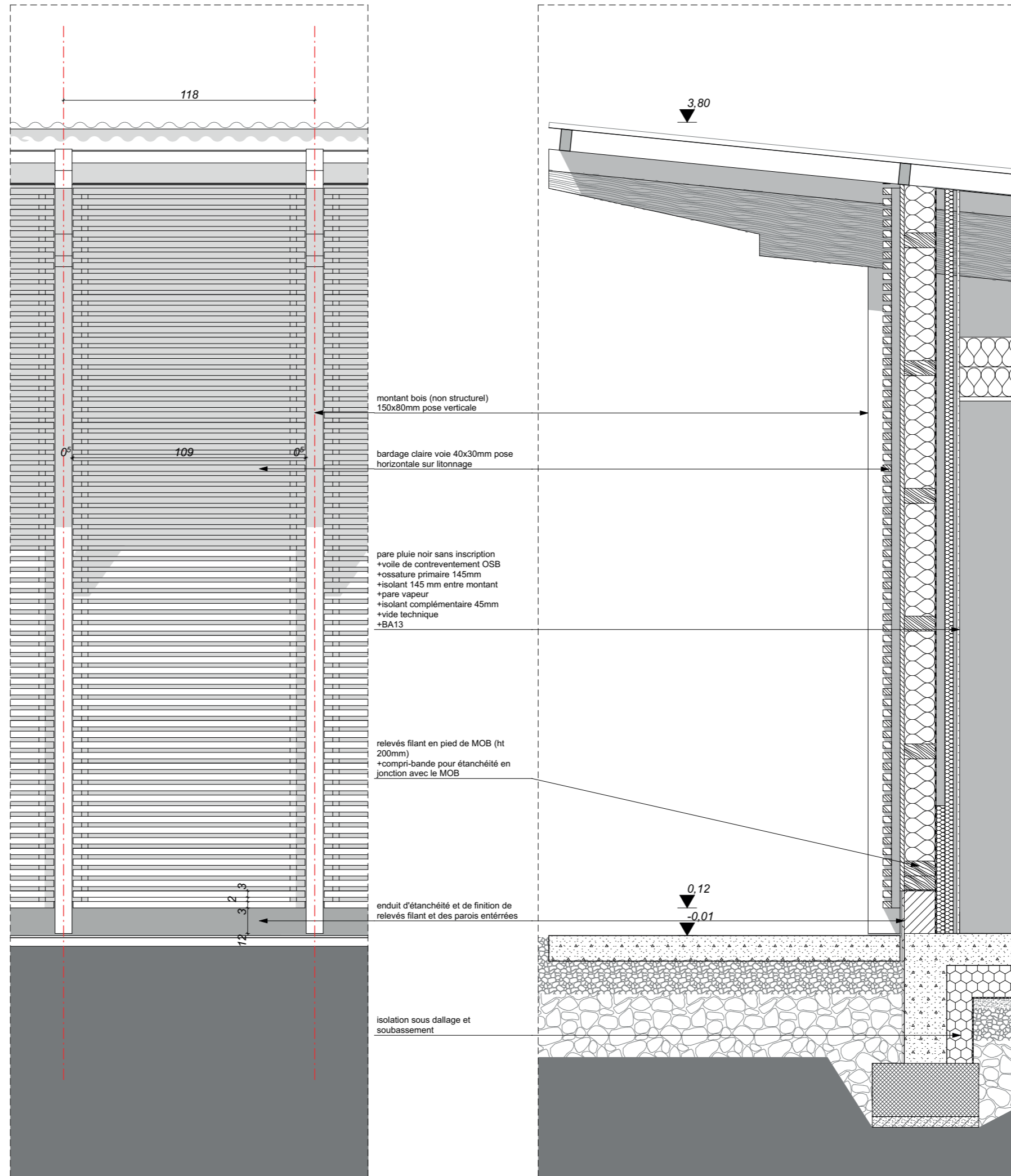
Détail sur partie courante 1/20 ème
