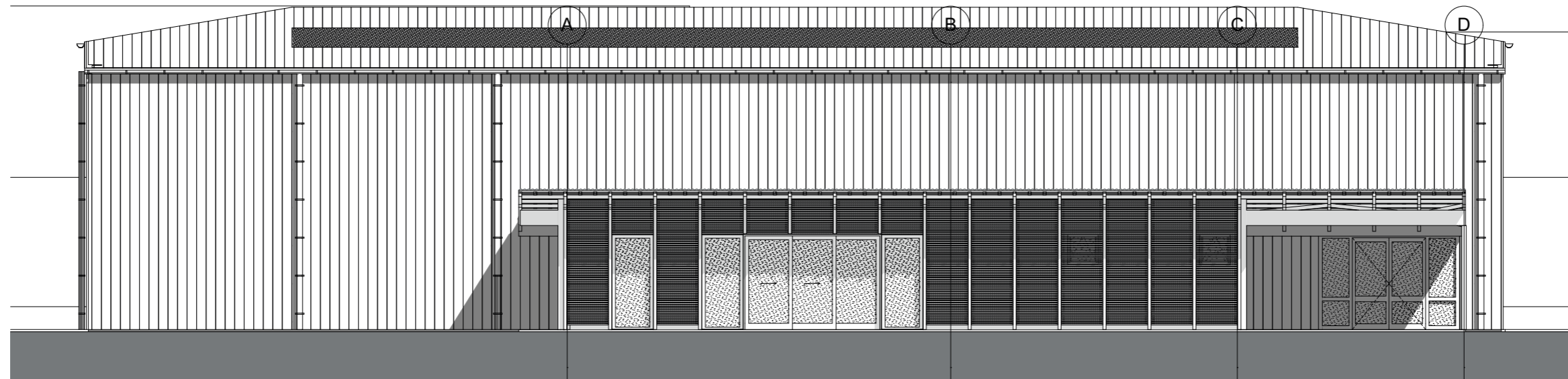
Façade Ouest 1/100 ème
