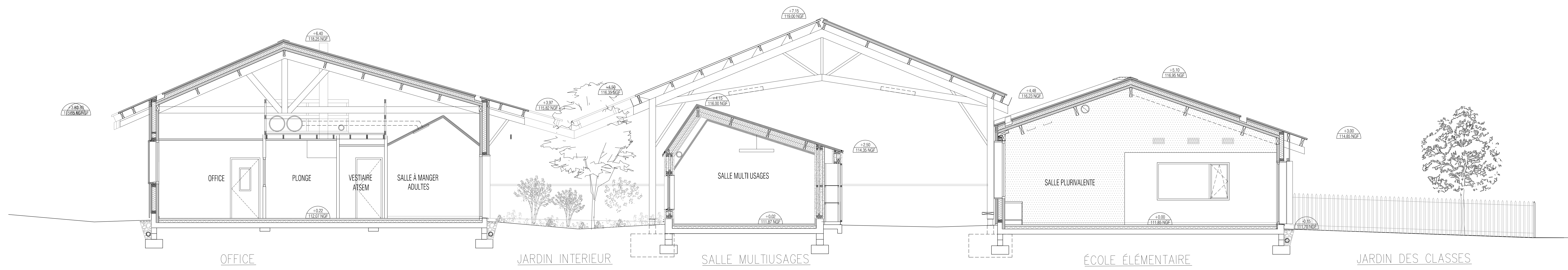
Coupe A-A
