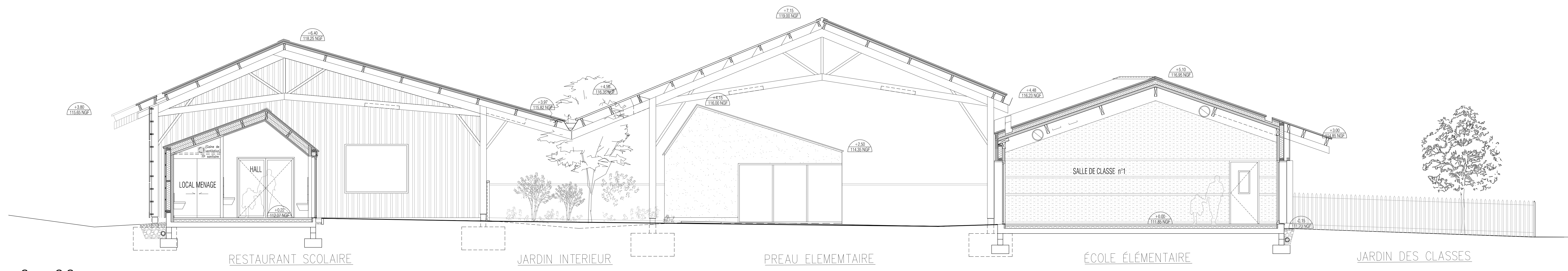
Coupe C-C
