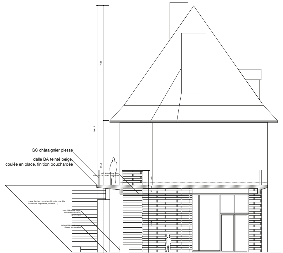
Coupe transversale de profil AA
