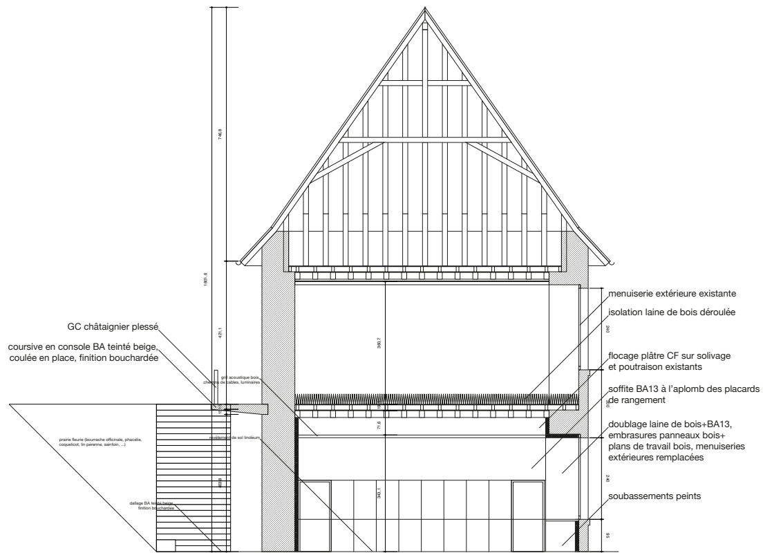
Coupe transversale de profil CC
